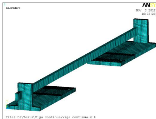
Figura 2. Modelo mallado de forma virtual de una viga de aluminio.
