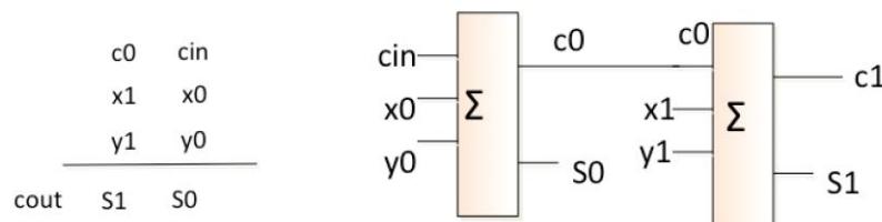
Figura 2. Aritmética y funcionamiento de un sumador de dos números binarios con dos bits.
