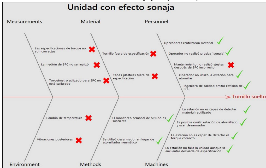
Figura 2. Posibles causas mediante diagrama de Ishikawa.
