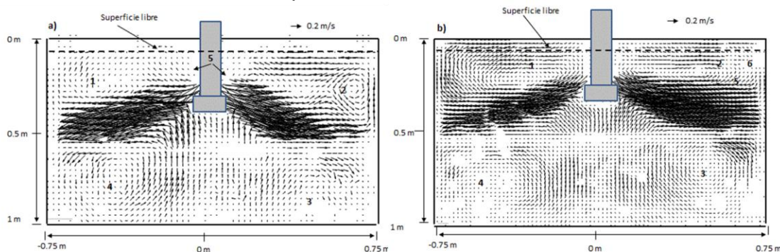
Figura 2. Campos de velocidad en el plano de simetría longitudinal del molde. a) Buza Sin Piscina (sp), b) Buza Con Piscina (cp).
