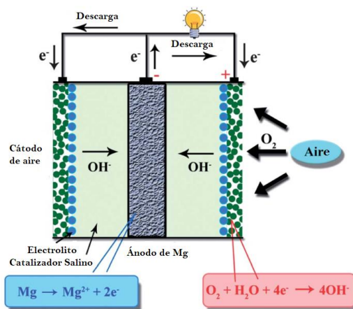
Figura 2: batería Mg-Aire
