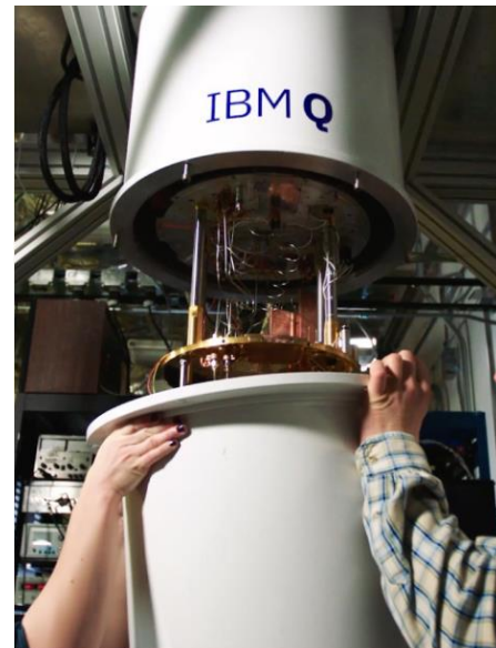
Figura 4: Procesador Cuántico.
