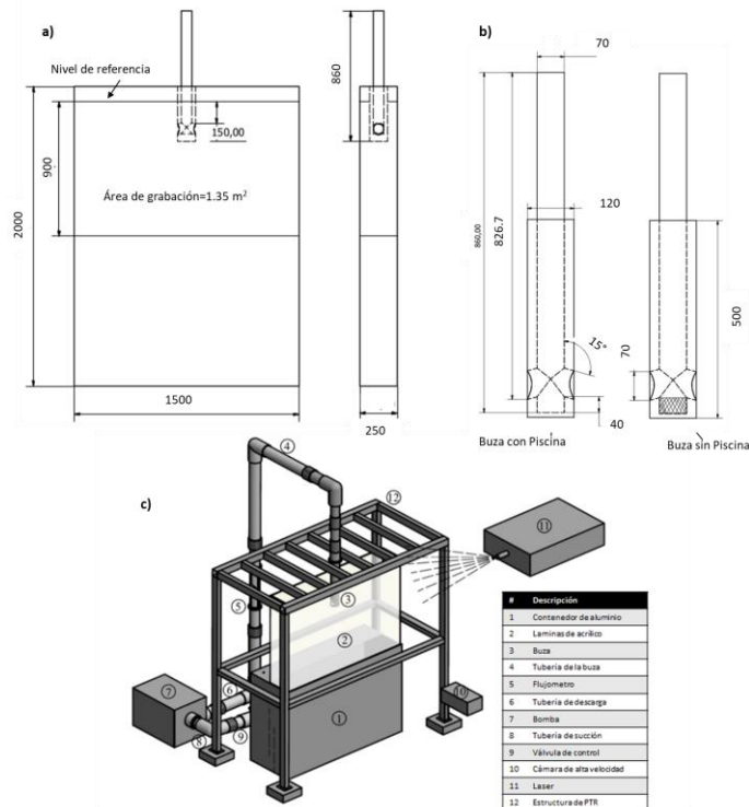
Figura 1. Dimensiones y esquema del arreglo experimental. a) Dimensiones del molde, b) Dimensiones de las buzas, c) Esquema de operación del arreglo experimental.
