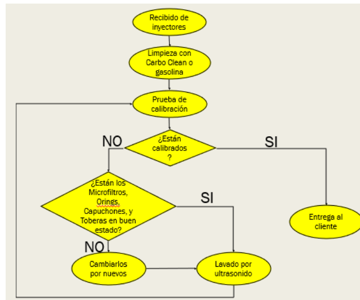
Figura 5. Diagrama de flujo de operaciones del método utilizado en el lavado por ultrasonido
