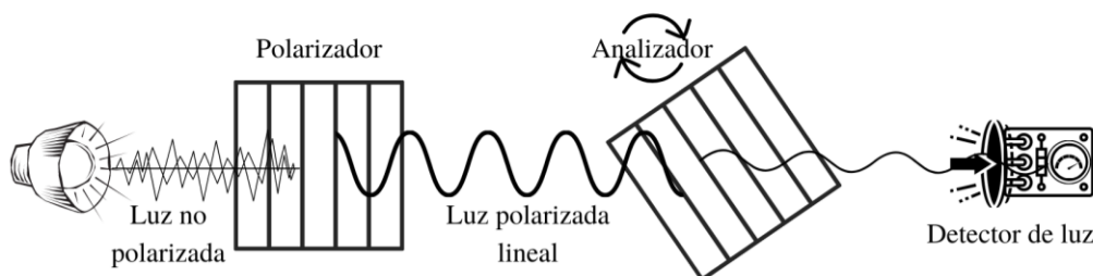
Figura 1. Esquema experimental para la medición de la ley de Malus.
