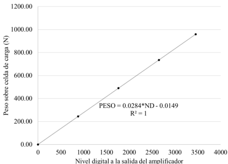
Figura 3. Curva de calibración de la celda de carga OMEGA LC703.
