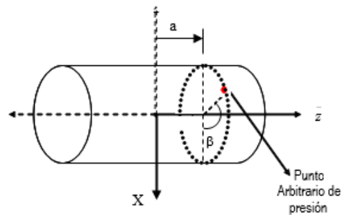
Figura 3. Ubicación del punto de presurización en el soporte. Notar que se definen los valores de las coordenadas axial y circunferencial ( a, \beta ) para especificar el punto en particular de inyección de lubricante.
