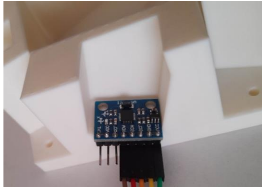
Figura 8 Ubicación de la IMU en prueba de medición del ángulo de 30°.
