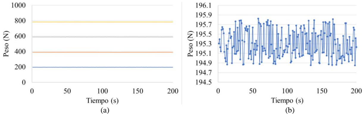
Figura 4. (a) Medición de prueba de validación de la celda de carga empleando 4 pesos distintos y (b) amplificación de la señal del peso registrada por el sistema de adquisición de datos para un objeto con peso de 195.11 N.
