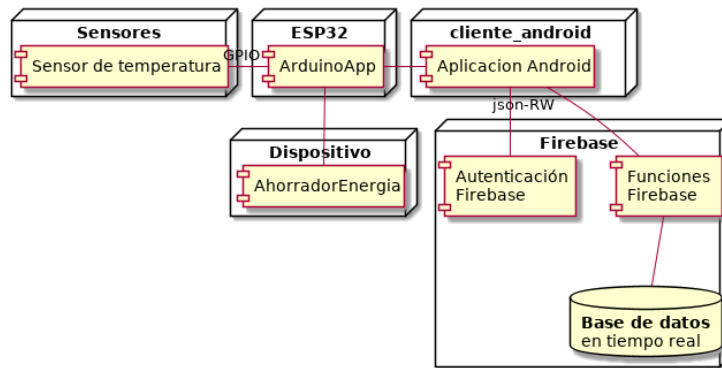
Figura 11: Despliegue de la aplicación
