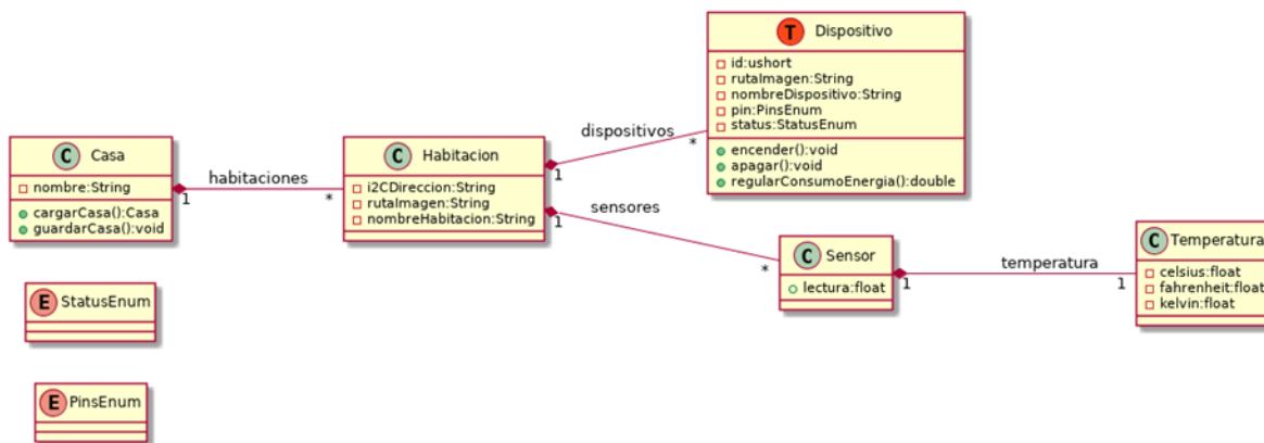
Figura 9: Diagrama de clases ejemplo
