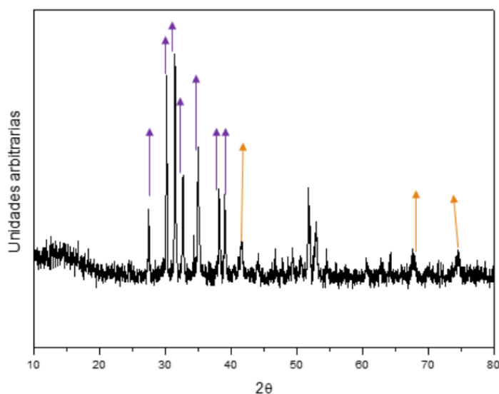
Figura 1. Difractograma de la reacción de coprecipitación de mineral de celestita con sulfato de ferroso. hexaferrita de estroncio (flecha morada). Óxido de hierro(flecha naranja)
