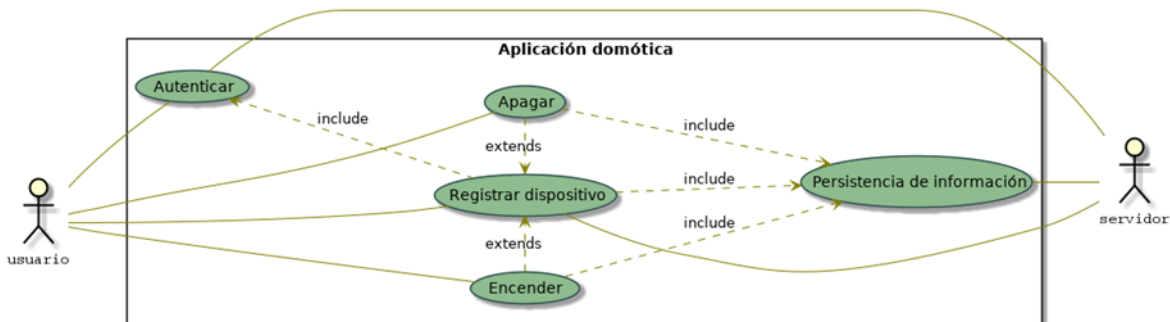
Figura 5: Ejemplo sencillo de diagrama de caso de uso
