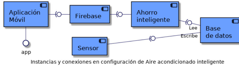
Figura 10: Diagrama de componentes ejemplo
