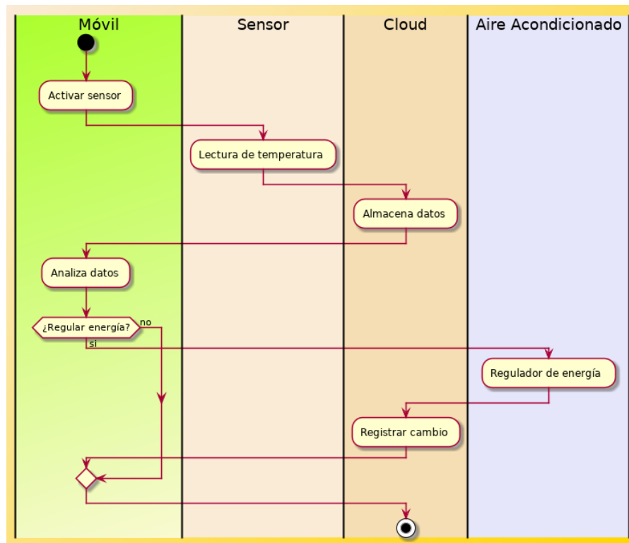
Figura 6: Diagrama de actividades ejemplo.
