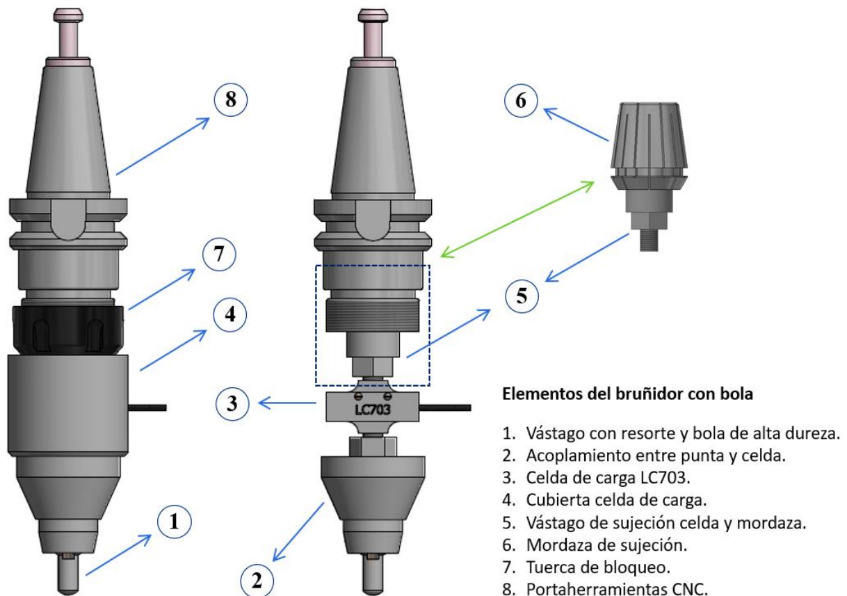
Figura 1. Diseño conceptual de prototipo de bruñidor mecánico con celda de carga.
