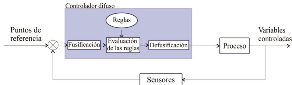
Figura 1. Sistema de control difuso.
