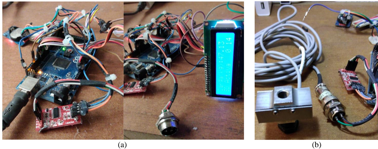
Figura 2. (a) Sistema de adquisición de datos para medir y registrar fuerza de bruñido y (b) celda de carga miniatura LC703 de OMEGA empleada en el proyecto de desarrollo de bruñidor con medición y registro digital de fuerza.
