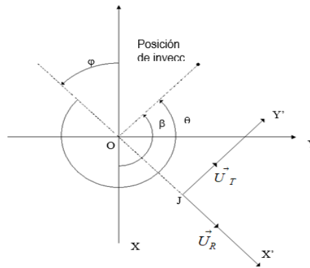
Figura 1. Sistemas de coordenadas: XOY-inmóvil, X'Y' móvil, "φ"-ángulo de equilibrio, "β" coordenada circunferencial de la posición de inyección en el sistema XOY.
