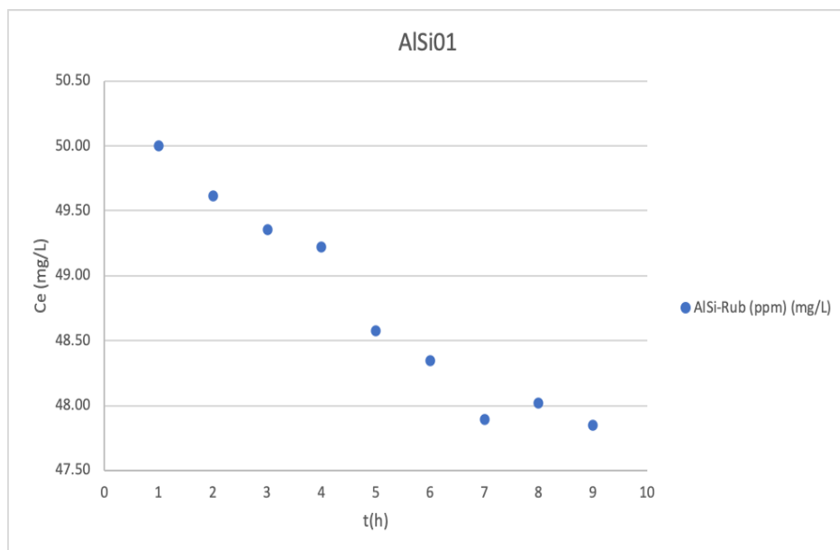
Figura 1. Cinética de sorción de cefepime sobre AlSi01
