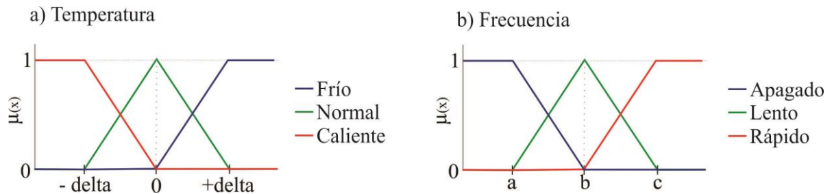
Figura 2. Funciones de membresía para las variables de entrada y salida del controlador.
