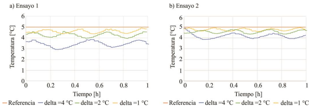
Figura 5. Comportamiento térmico del refrigerador.
