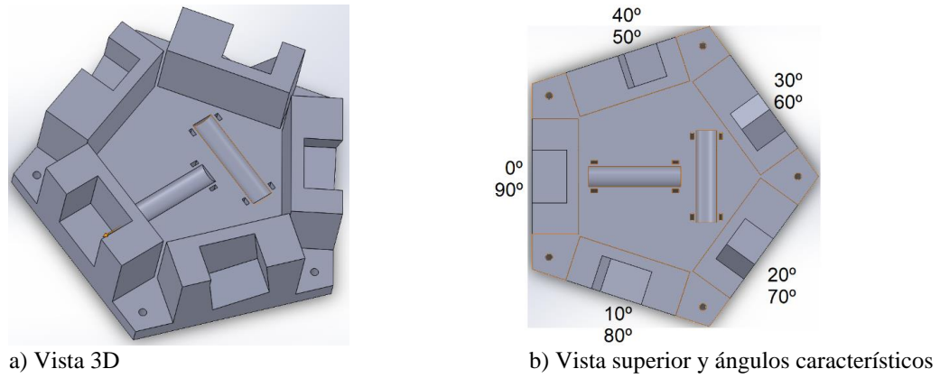
Figura 5. Diseño Impreso del sistema.
