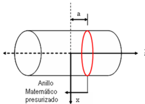
Figura 2. Posición axial de alimentación de lubricante, notar que a una distancia "a" del centro del soporte se presenta la inyección, pero en forma circular (anillo presurizado), además que en esta situación no se especifica la posición circunferencial de presurización.
