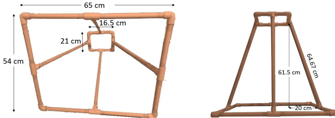
Figura 1 Estructura física.
