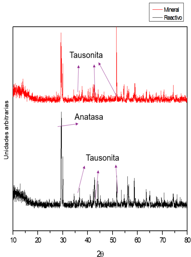
Figura 2. Difractograma que muestra las fases presentes de la reacción entre carbonato de estroncio y óxido de titanio grado reactivo y mineral a una temperatura de 800^\circ\text{C} y 8 horas de permanencia
