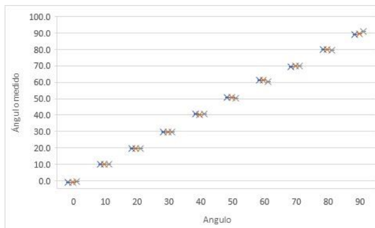
Figura 9 Lectura final de ángulos con sistema calibrado.
