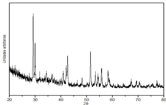
Figura 1. Difractograma del Mineral de celestita carbonatado
