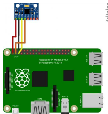
Figura 2 Conexión entre Raspberry Pi y MPU6050
