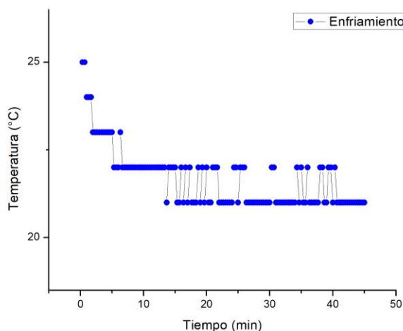
Figura 3 Gráfica correspondiente a la temperatura de enfriamiento obtenida dentro del recipiente.
