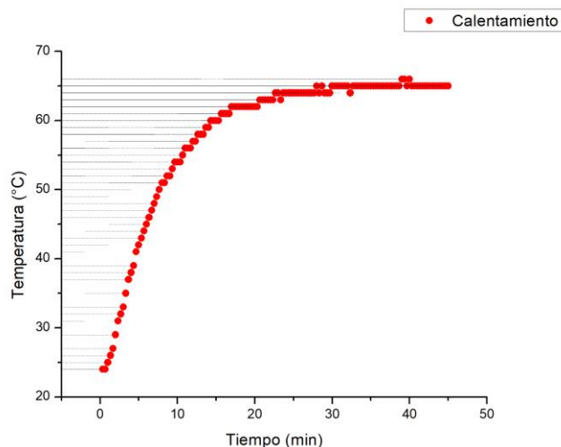
Figura 4 Gráfica correspondiente a la temperatura de calentamiento obtenida dentro del recipiente.
