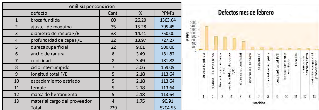
Figura 13. Principales defectos de línea 4 en el mes de febrero
