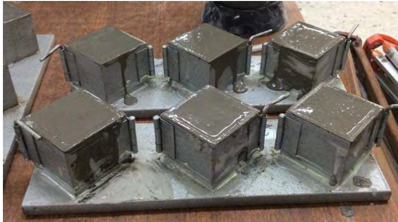
Figura 4. Ejemplos de cubos de morteros con la mezcla diseñada.
