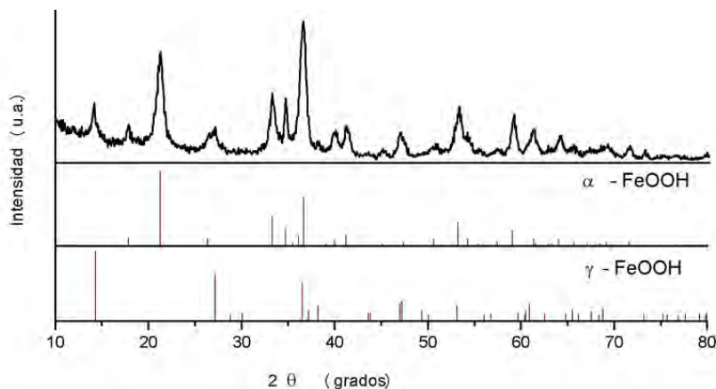
Figura 2. Diffractograma de la goetita sintetizada; patrón de goetita (PDF 96-901.0407) y patrón de lepidocrocita (PDF 96-900-9155).
