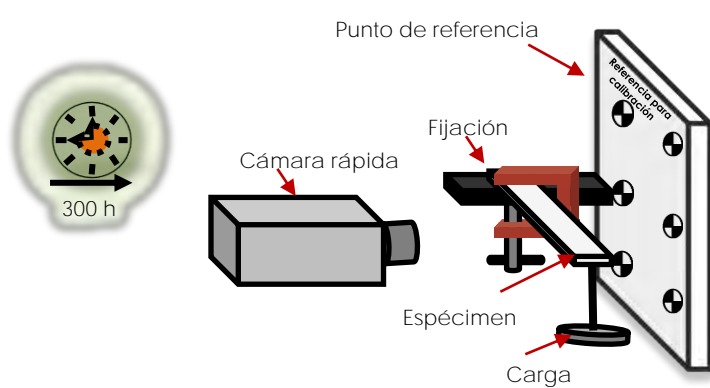
Figura 2. Modelo experimental del método propuesto para pruebas de fluencia lenta.
