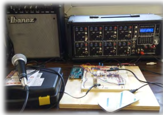
Figura 6: Sistema real.
