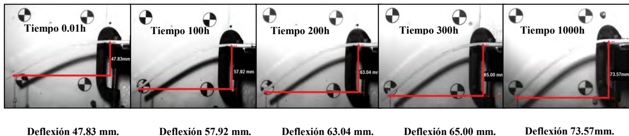
Figura 5. Visualización de la deflexión en espécimen de ABS con una carga 5.11 N.
