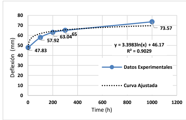
Figura 6. Curva ajustada y real de fluencia lenta ABS con una carga de 5.11 N.
