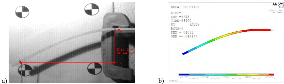
Figura 10. Prueba de fluencia lenta con una carga de 5.6N a) experimental b) Análisis numérico.
