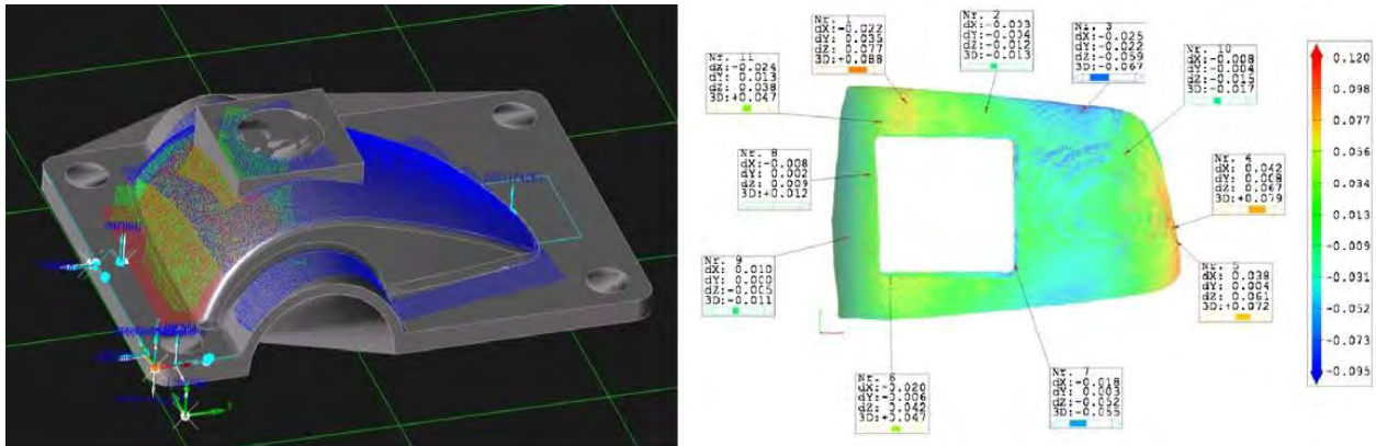
Figura 1. Imagen de un herramental reconstruido en 3D (Haibin y Pean-Pierre 2012).
