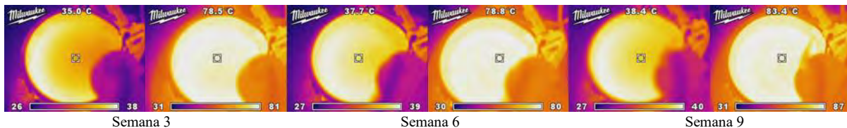
Figura 11. Imágenes con cámara infrarroja de la semana 3, 6 y 9, con la resistencia a 40°C y 100°C, respectivamente.
