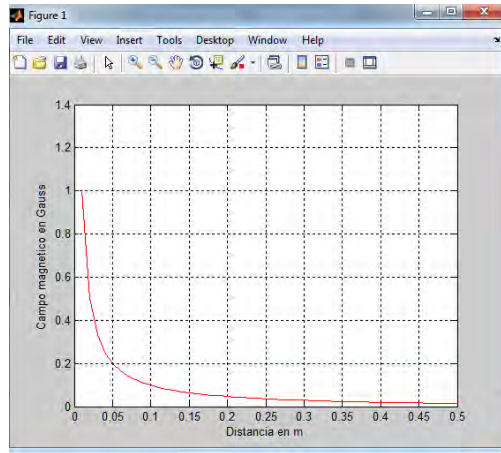
Figura5. Grafica de comportamiento del campo magnético
