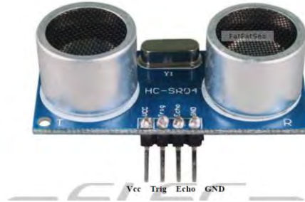
Figura 3. Sensor ultrasónico
