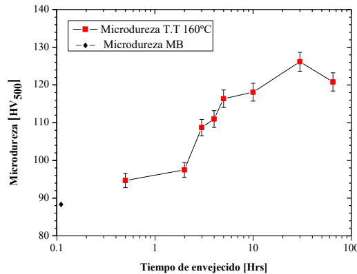
Figura 5.- Curva de endurecimiento de la aleación A356 envejecida a 160°C de 0.5 a 65 hrs.
