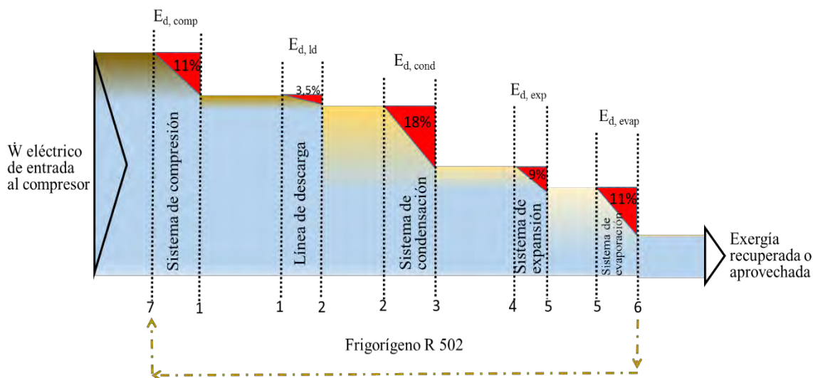
Figura 2. Diagrama de Grassman del sistema de congelación.
