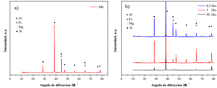
Figura 4.- Patrones de difracción de la aleación de Al A356, tratada térmicamente.
