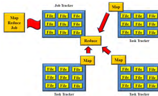
Figura 1. Esquema de componentes del framework MapReduce Fuente: (Summit, 2012)
