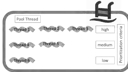
Figura No. 2. Thread Pools para priorización de tareas
