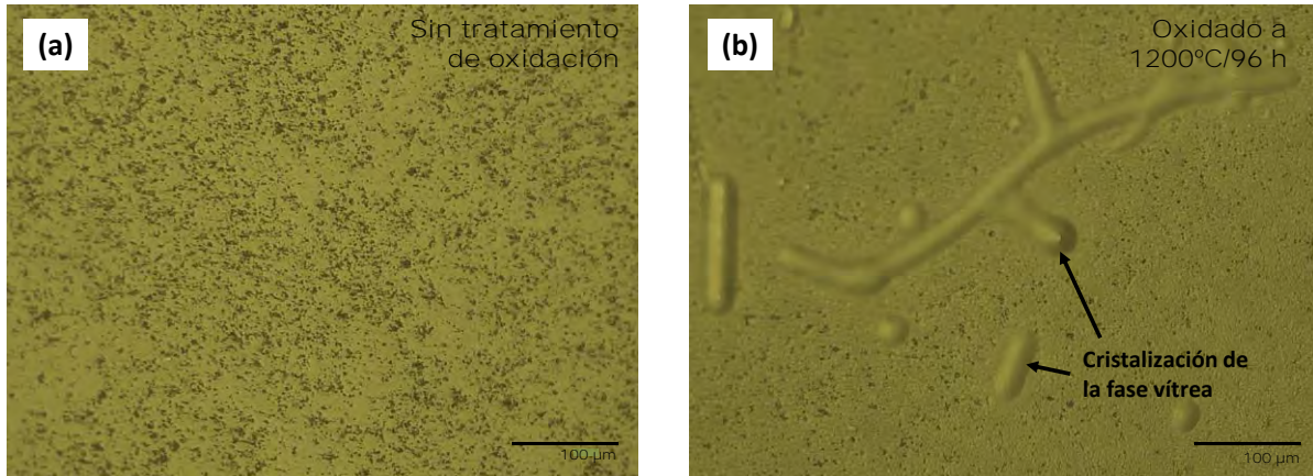
Figura 3. Micrografías por microscopía óptica de la superficie de los cerámicos de \text{Si}_3\text{N}_4 -4 antes y después del proceso de oxidación a temperatura elevada: (a) sinterizado a 1500^\circ\text{C}/5 min y (b) Oxidado a 1200^\circ\text{C}/96 h.
