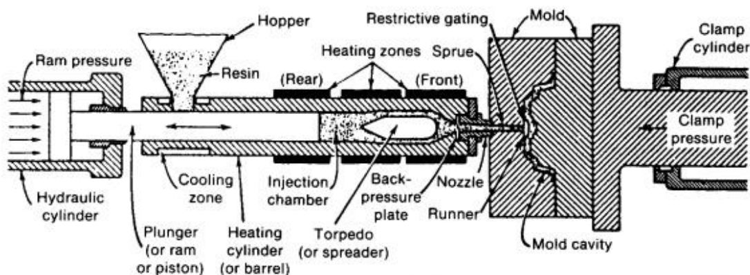
Ilustración 1: Proceso de inyección de plástico
