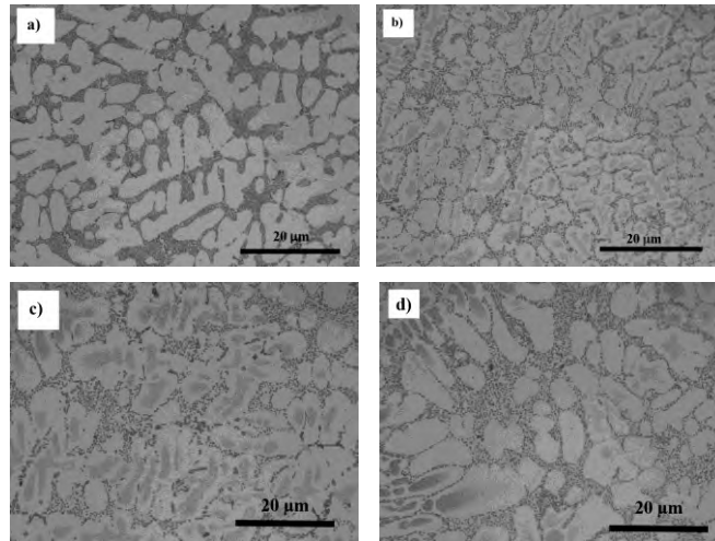
Figura 2.- a) Aleación A356 sin tratamiento térmico, b) muestra envejecida a 160°C durante 0.5 hrs, c) muestra envejecida a 160°C durante 3 hrs y d) muestra envejecida a 160°C durante 30 hrs.
