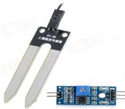
Figura 1. Sensor FC-28, para el control de humedad en el suelo.
