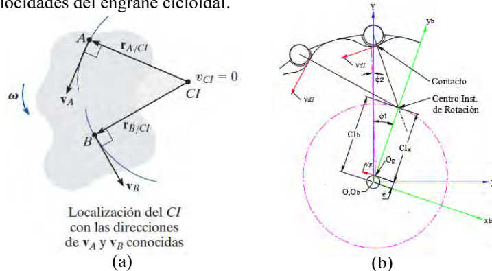
Figura 4. Centro instantáneo de rotación: (a) definición; (b) relaciones geométricas del reductor
