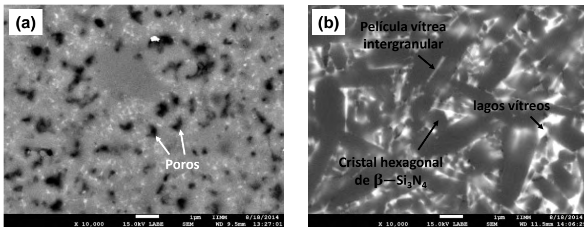
Figura 2. Micrografías por FESEM de la superficie pulida de los cerámicos de \text{Si}_3\text{N}_4 producidos a partir de dos composiciones distintas: (a) \text{Si}_3\text{N}_4 -4 y (b) \text{Si}_3\text{N}_4 -12.
