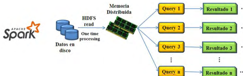
Figura 5. Operación interactiva en RDD Spark Fuente: (Esteso, 2017).
