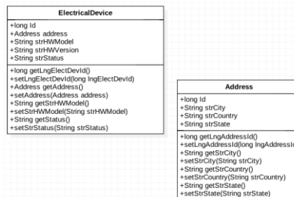
Figura No. 3 Ejemplo de anidamiento de objetos
