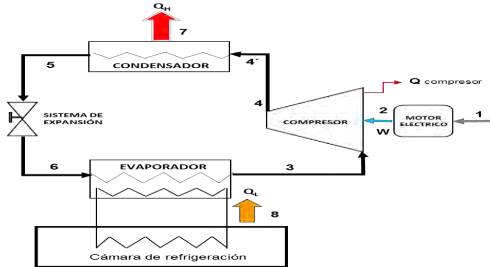
Figura 1. Ciclo básico de refrigeración por compresión de vapor. Adaptado de Cengel y Boles, (2013).
