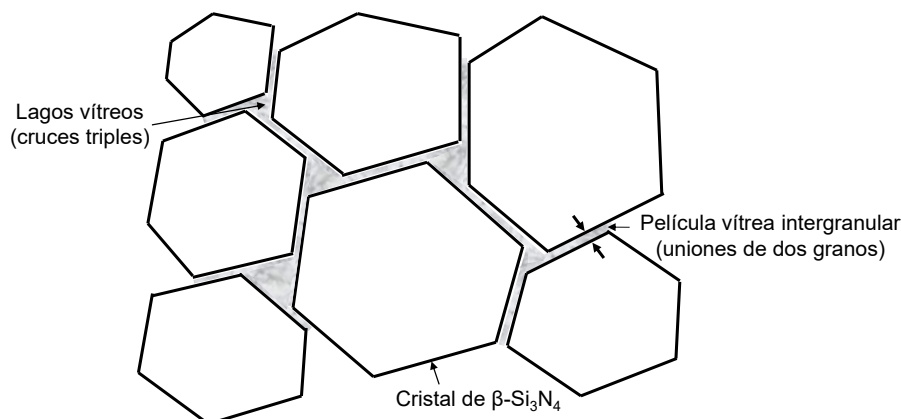
Figura 1. Esquema representativo de la microestructura en cerámicos de \beta - \text{Si}_3\text{N}_4 .
