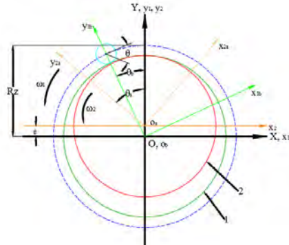
Figura 1. Sistema de Coordenadas y diámetros primitivos de la rueda de rodillos y del engrane cicloidal
