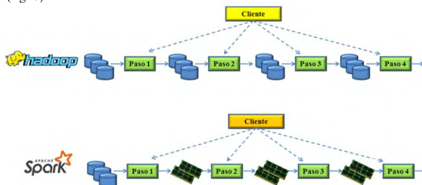
Figura 6. Operaciones y procesos de Hadoop y Spark Fuente: (Wui3, 2017)
