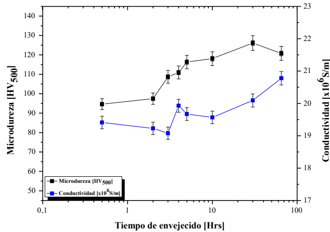
Figura 6.- Conductividad medida en la aleación A356 envejecida a 160°C
