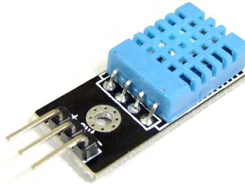
Fig. 2 Sensor DHT11, para el control de temperatura en el invernadero.
