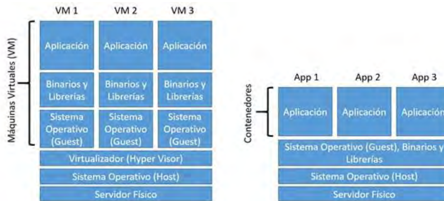
Máquinas Virtuales versus Contenedores
