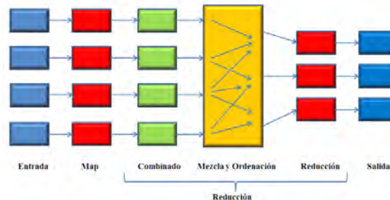
Figura 2. Proceso de Procesamiento de Hadoop y MapReduce Fuente: (Summit, 2012)
