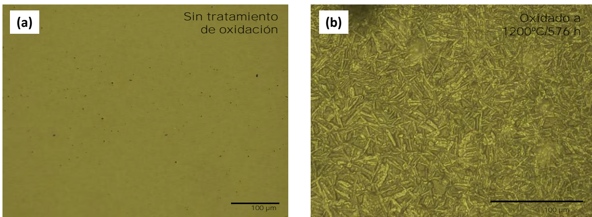
Figura 4. Micrografías por microscopía óptica de la superficie de los cerámicos de \text{Si}_3\text{N}_4 -12 antes y después del proceso de oxidación a temperatura elevada: (a) sinterizado a 1500^\circ\text{C}/5 min y (b) Oxidado a 1200^\circ\text{C}/576 h.
