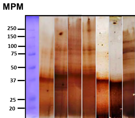
Figura 3. Fosfoproteoma de pulmón de ratones infectados con Yersinia pseudotuberculosis . El extracto de proteínas fosforiladas se sometió a electroforesis SDS-PAGE al 10%, después del corrimiento se procedió a teñir con plata
