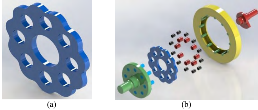
Figura 2. Reductor cicloidal: (a) Engrane cicloidal; (b) vista explosionada
