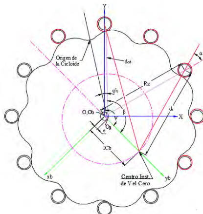
Figura 5. Angulo de presión y ángulo de contacto
