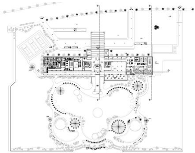
Figura 6. Planta arquitectónica de conjunto
