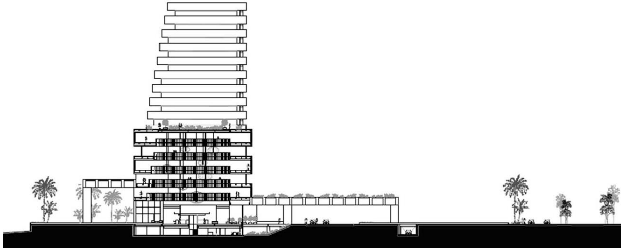
Figura 9. Corte transversal
