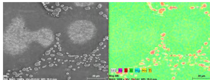
Figura 3.- Mapeo realizado a la muestra 6 envejecida 3 hrs.
