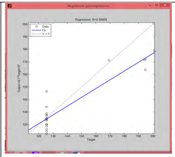
Figura 4. Gráfica de correlación de dureza
