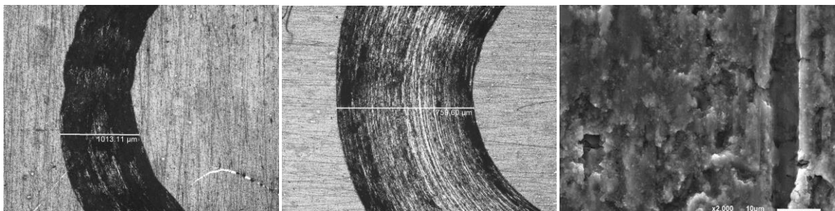
Figura 3 Imágenes ópticas de la huella de desgaste de la aleación AZ91E a 1 N a una velocidad de deslizamiento de a) 5cm/s, b) 15cm/s, c) Imagen MEB (15cm/s)
