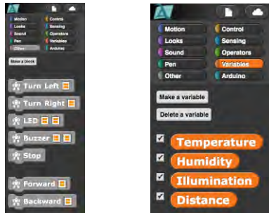
Figura 1: Nuevos bloques y variables en Snap4Arduino.
