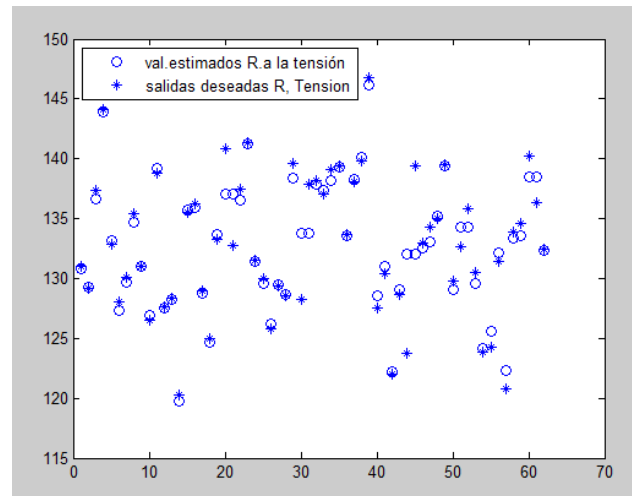
Figura 7 Valores estimados vs deseados del factor R. a la tensión
