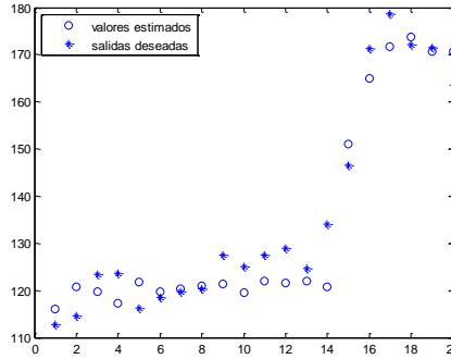
Figura 5. Valores estimados vs deseados dureza
