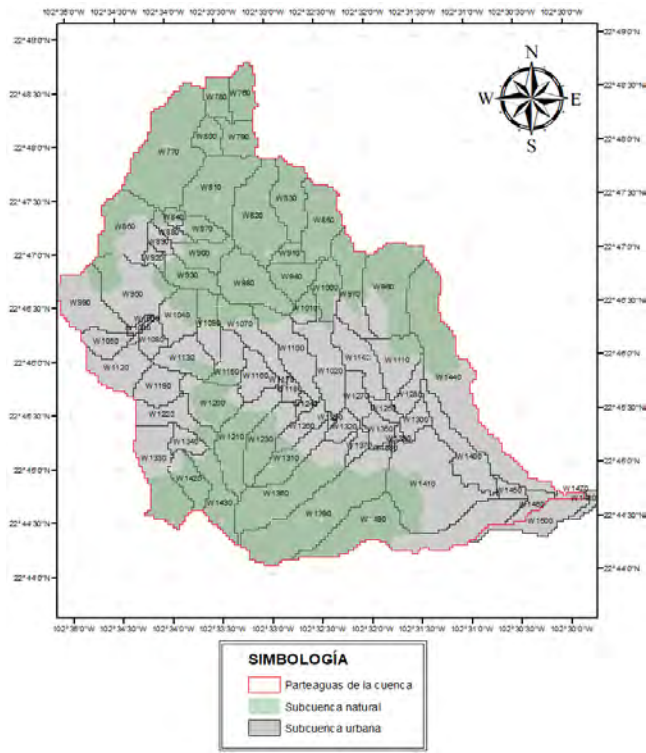
Figura 2. Subcuencas generadas con el software Arc Hydro
