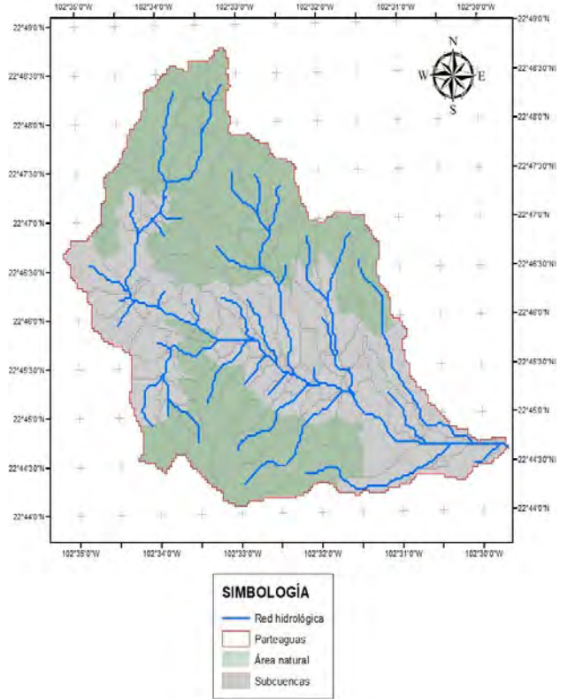
Figura 3. Red hidrológica de la cuenca
