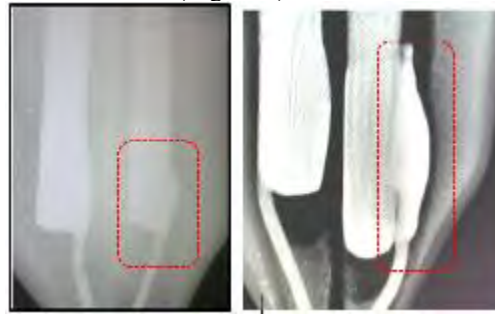
Figura 2. Defectos de soldadura en proceso manual
