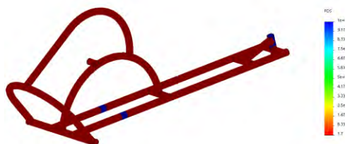
Figura 6. Distribución del factor de seguridad.
