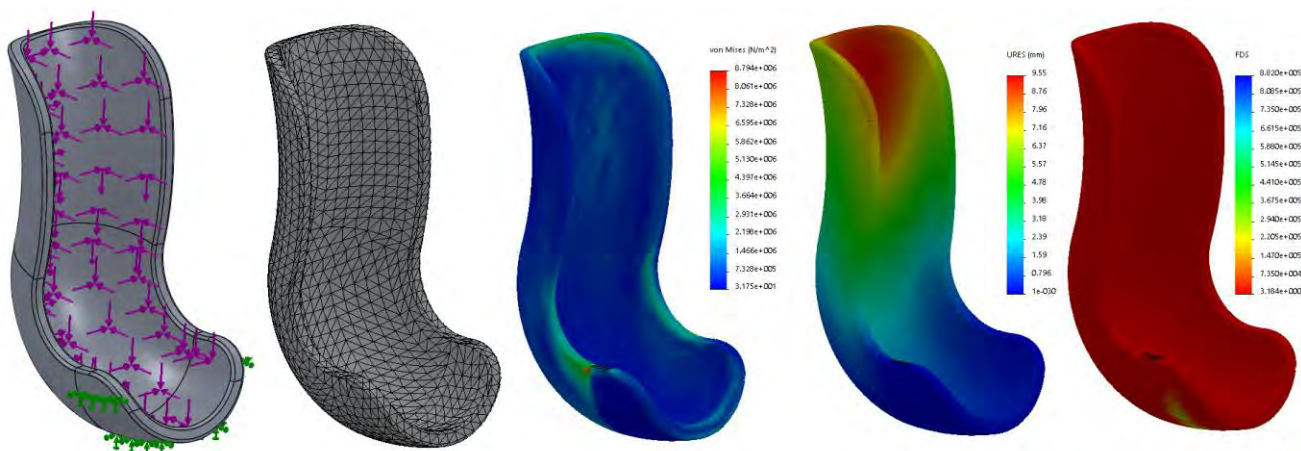
Figura 7. Análisis estático de asiento en material ABS
