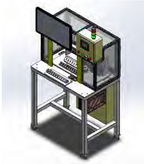
Figura 3. Diseño mecánico en programa Solid Works
