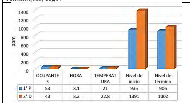
Figura 6. Niveles de CO 2 en la Escuela Secundaria Técnica No. 13 Antonio Soto Gama de Atitalaquia, Hgo.
