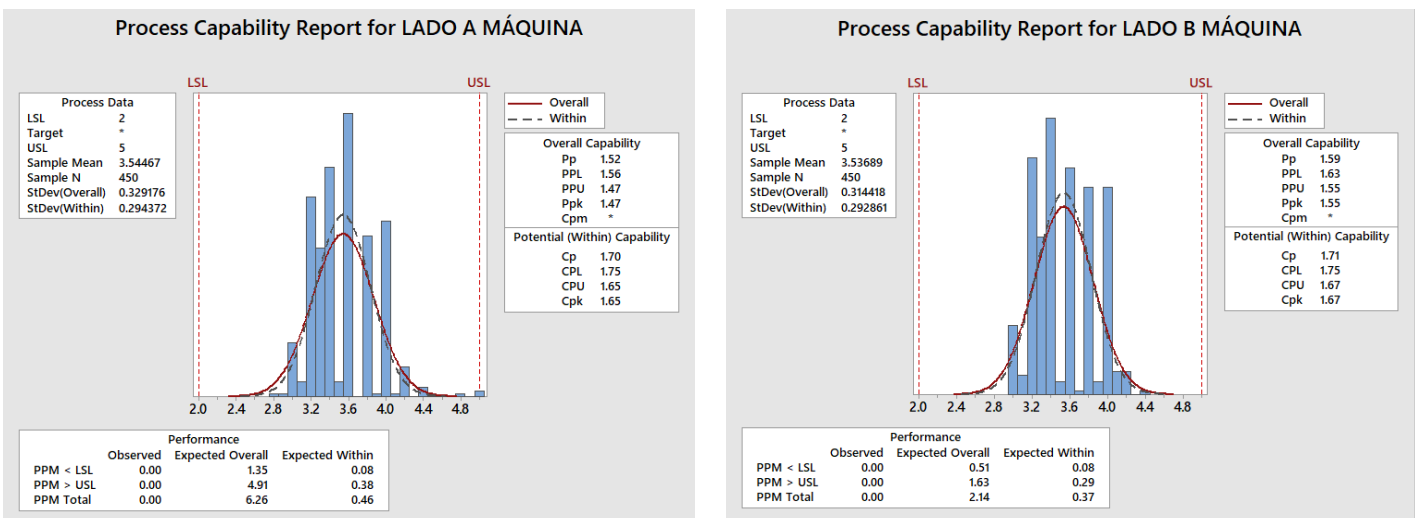
Figura 9. Cálculo de PPK para proceso semi automático
