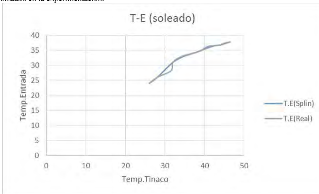
Figura (2). Simulación de la reconstrucción de datos para la temperatura de entrada en salida del tanque de almacenamiento
