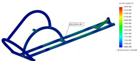
Figura 4. Mapa de distribución de esfuerzos de Von mises
