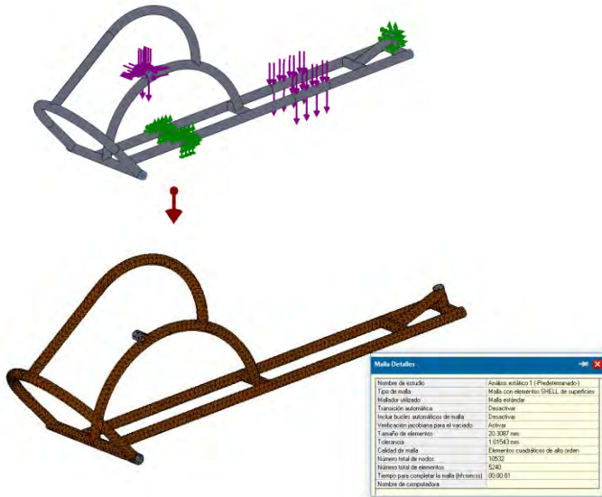
Figura 2. Sujeciones y cargas externas
