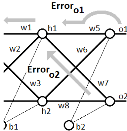
Fig. Propagación del error en la red neuronal
