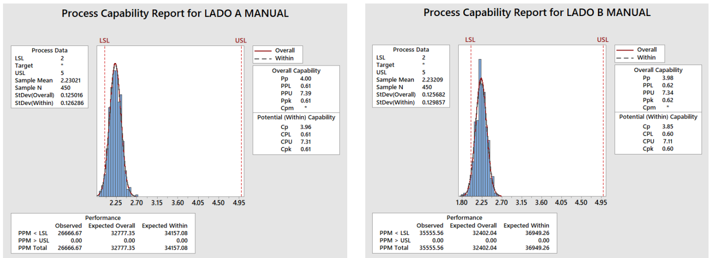
Figura 8. Cálculo de PPK para proceso manual.
