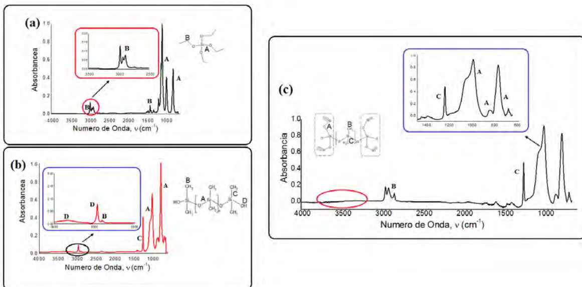
Figura 2. Espectroscopia de Infrarrojo (a) Precursor cerámico TEOS (b) Elastómero PDMS (c) Céramico híbrido ORMOCER-UPIIG
