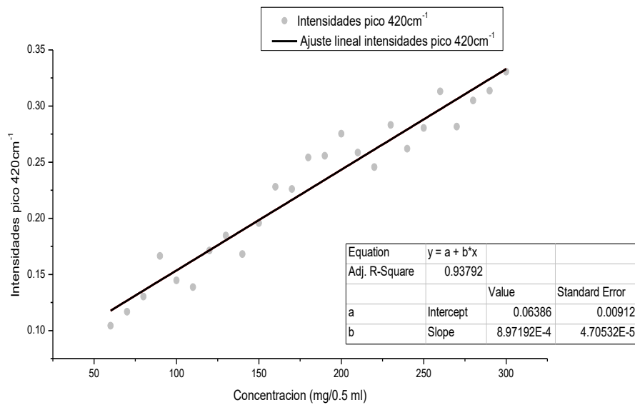
Figure 2. Relación entre la intensidad Raman y la concentración de dextrosa en el pico ubicado en 420\text{ cm}^{-1}
