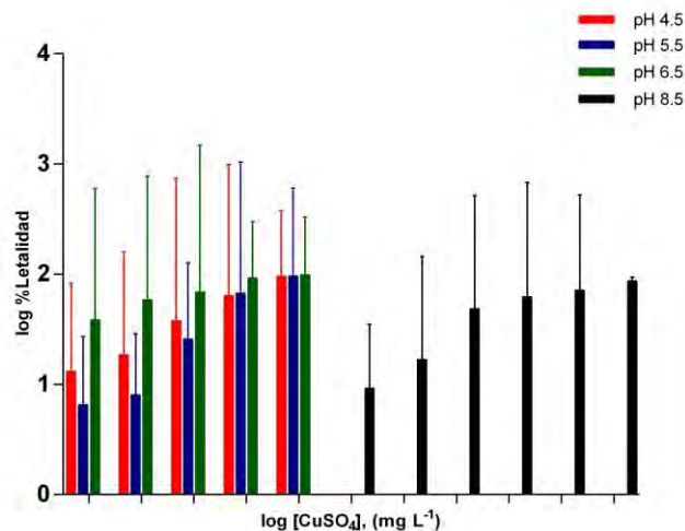
Gráfico 2 Comparación de las respuestas de A. franciscana CL 50(24) a los diferentes pH
