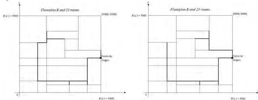
Figura 4. Corredores en un rectángulo R con 23 rectángulos
