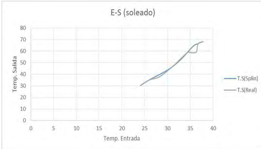
Figura (3). Simulación de la reconstrucción de base de datos
