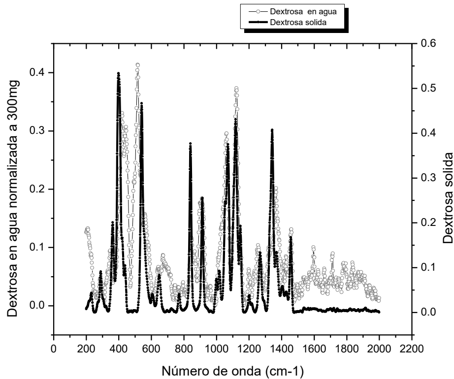
Figure 1. Forma de línea Raman de dextrosa solida vs 300 mg de dextrosa en agua
