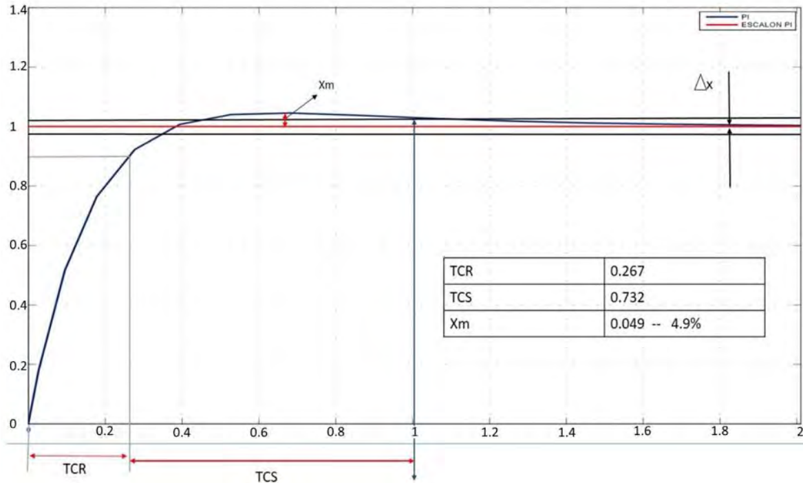
Figura (2) Imagen de la gráfica utilizada para la evaluación de controlador PI.
