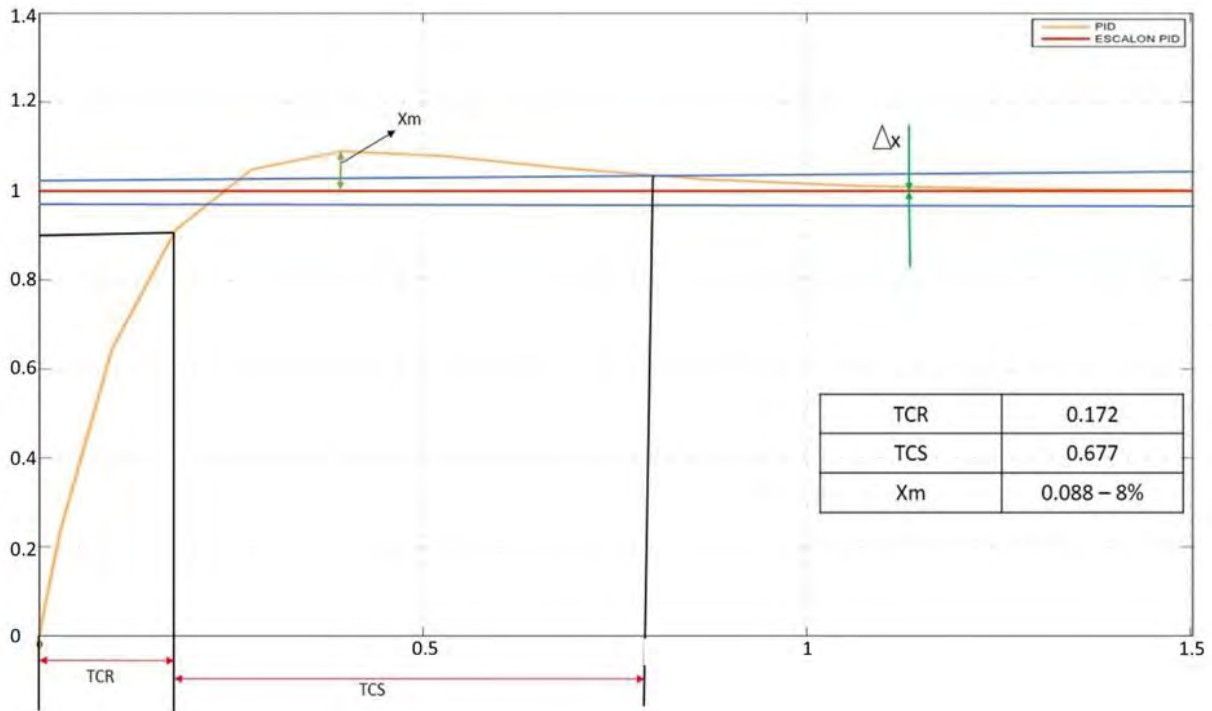
Figura (1) Imagen de la gráfica utilizada para el análisis de los controlador PID.
