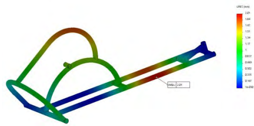
Figura 5. Desplazamientos resultantes
