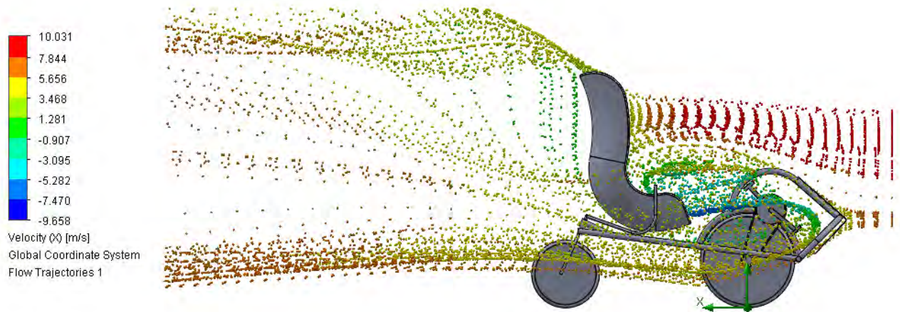
Figura 9. Análisis Aerodinámico
