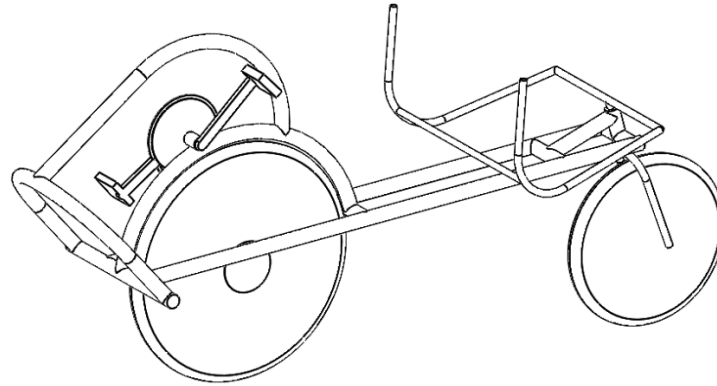
Figura 8. Detalle de sistema de dirección trasero tipo palanca
