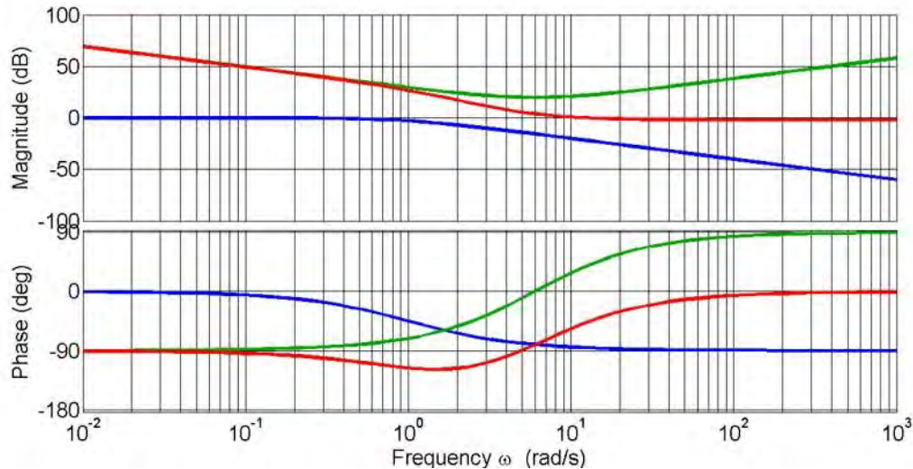
Figura (3) Imagen BODE en la frecuencia de un controlador PID
