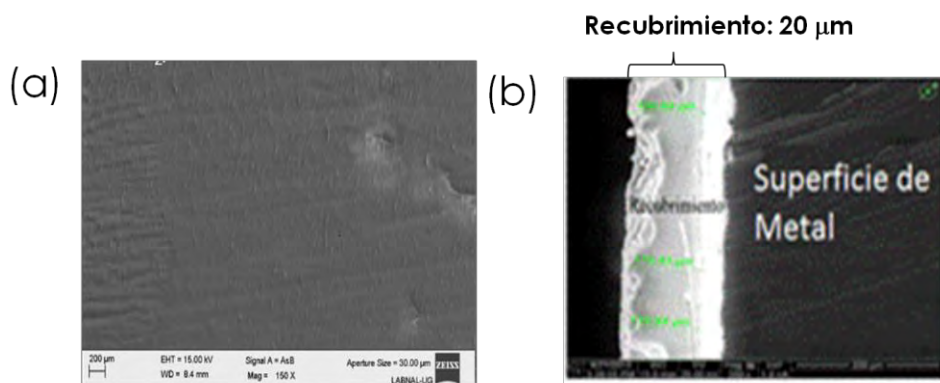
Figura 3. MEB de ORMOCER-UPIIG depositado sobre Al-6061 (a) vista frontal (b) vista lateral Determinación de Conductividad Térmica
