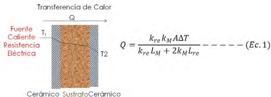
Figura 1. Sistema empleado para la determinación de la conductividad térmica
