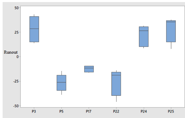
Figura 1. Diagrama de caja de la piezas elegidas contra sus mediciones.
