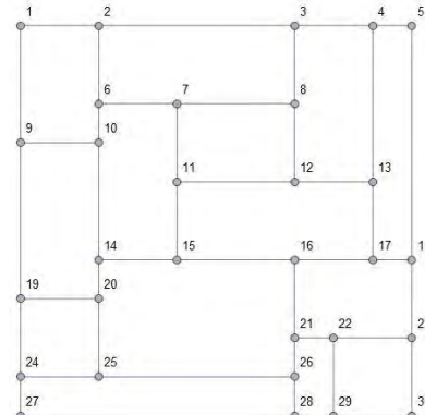
Figura 6. Grafo Acíclico Conexo Ponderado
