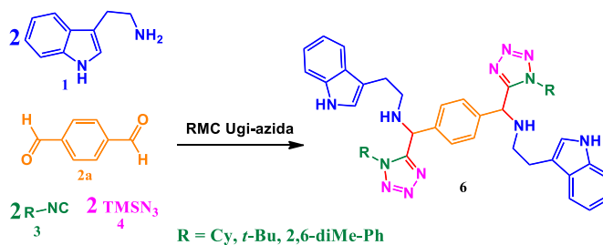
Figura 3. Esquema general de síntesis.
