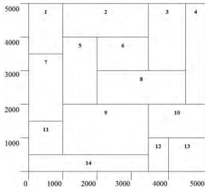
Figura 5. Instancia Geométrica Rectángulo
