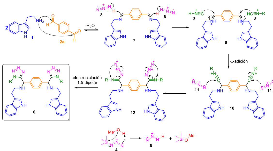
Figura 4. Mecanismo de RMC Ugi-azida.
