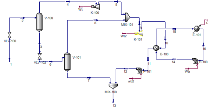
Figura 3: Sistema Geotérmico de Doble Flash
