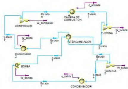
Figura 4: Diagrama HYSYS Ciclo Combinado
