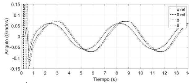
Figura 6. Ángulos de \theta y \phi deseados con técnicas de Lyapunov
