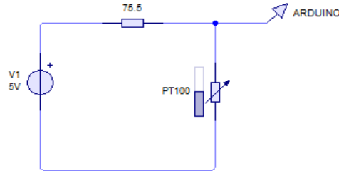
Figura 1 Resistencia
