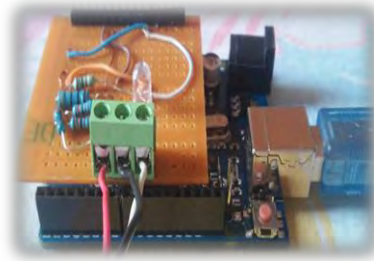
Figura 2 Placa auxiliar
