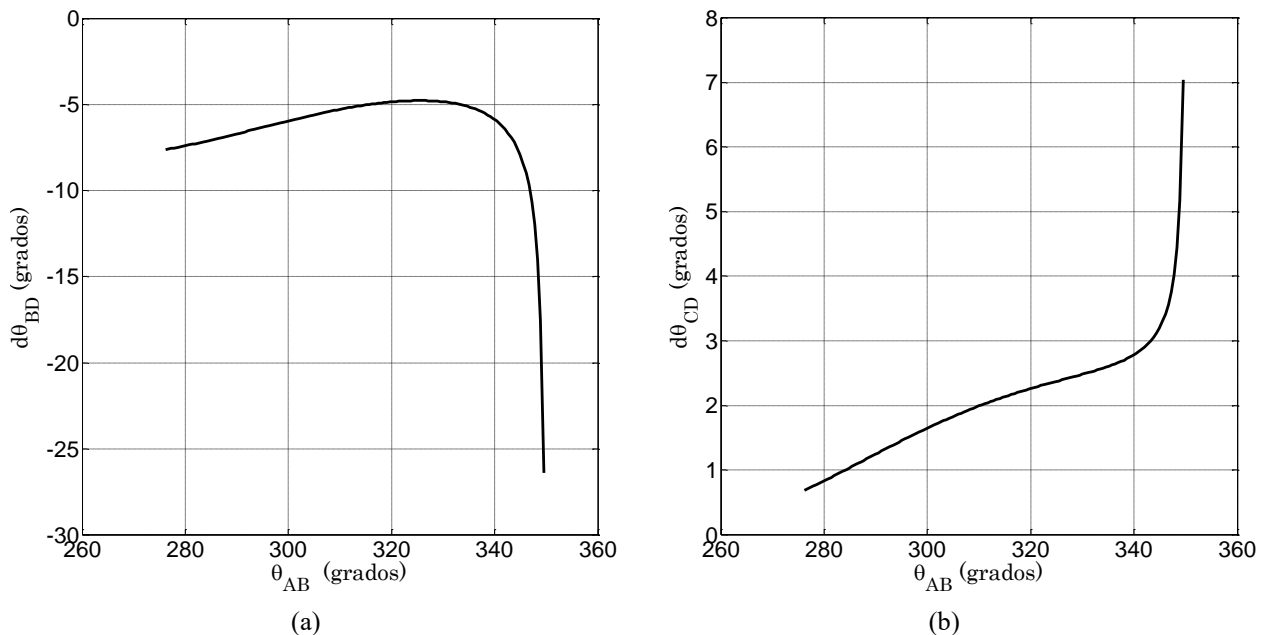
(a) (b) Figura 4. Evolución de los ángulos \theta_{BD} y \theta_{CD} para una variación de las barras de 0.5 mm.
