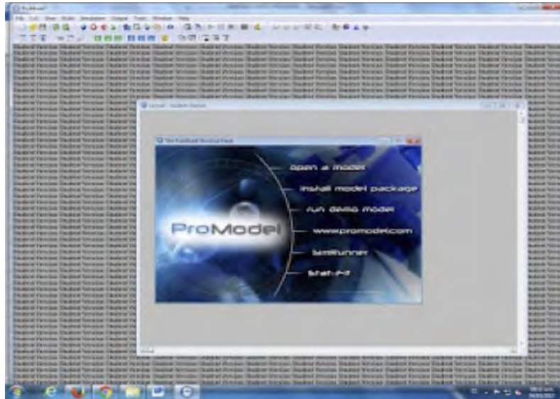
Figura 1. ProModel
