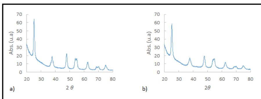
Figura 1. Difractogramas de rayos-x. a) \text{TiO}_2 RL, b) \text{TiO}_2\text{-ZrO}_2 RL
