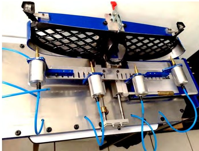
Figura 8. Prototipo físico del Checking Fixture.
