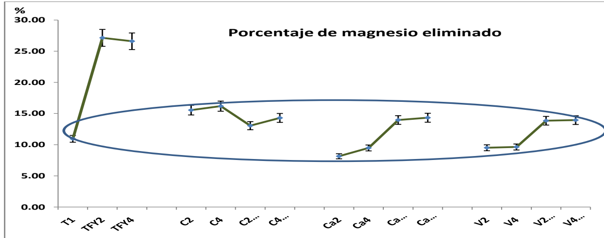
Figura 2. Porcentajes de reducción final de magnesio con diferentes tratamientos
