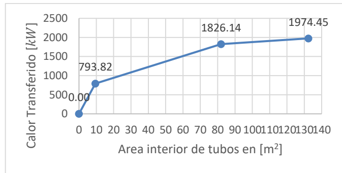
Figura 3.- Grafica de relación entre el área de transferencia y el calor transferido
