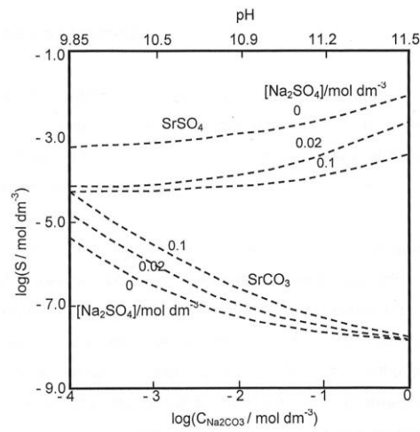
Figura 4. Solubilidad entre la Celestita sulfato de estroncio y el carbonato de estroncio en funcion de la concentracion del carbonato de sodio y el pH a 25°C
