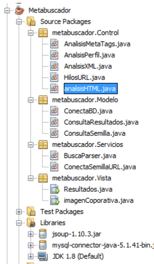
Figura 3. Paquete en JAVA del proyecto
