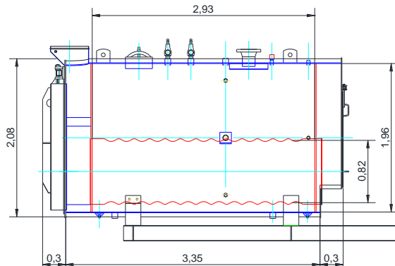
Figura 2.- Plano de Caldera vista lateral exterior y longitud
