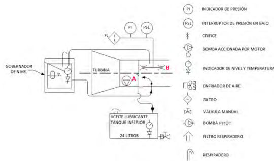
Figura 3. Sistema de lubricación y enfriamiento de una turbina. (GREEN-ER FIM UMSNH s.f.)
