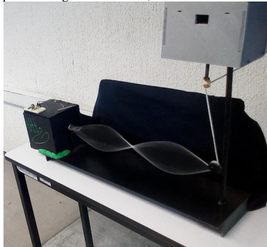
Figura 5. Dinamómetro digital montado en equipo de ondas estacionarias. Fuente elaboración propia.
