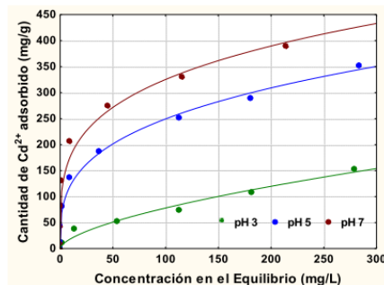
Figura 3. Isotermas de adsorción del material MAM ajustadas al modelo Freundlich.
