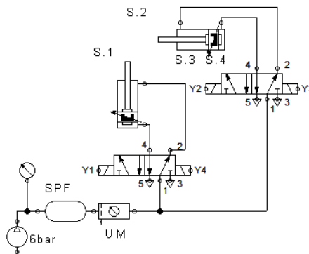
Figura 23 Circuito neumático
