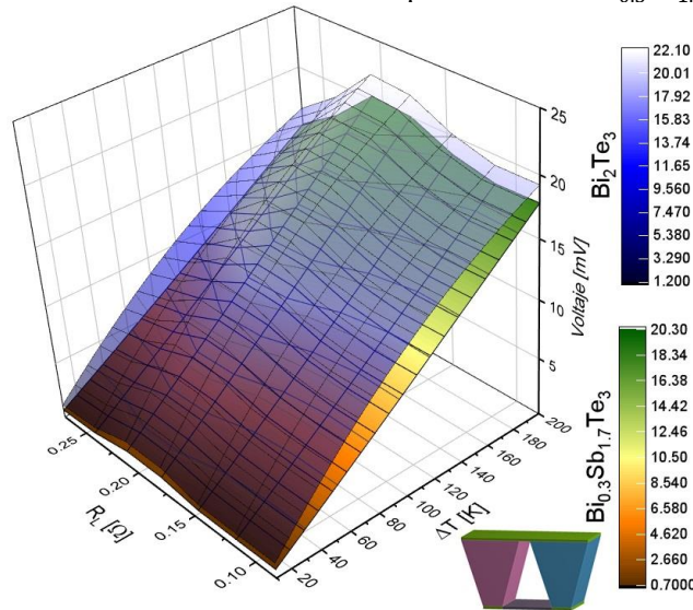
Figura 5. Voltaje de Salida en función de Resistencia de Carga ( R_L ) y diferencia de Temperatura ( \Delta T ) para un MTEG con termoelementos trapezoidales.
