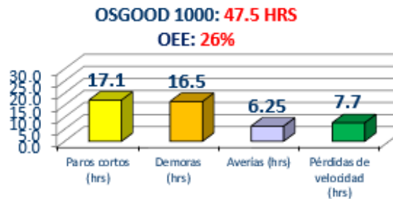
Figura 2. Eficacia global de la maquina
