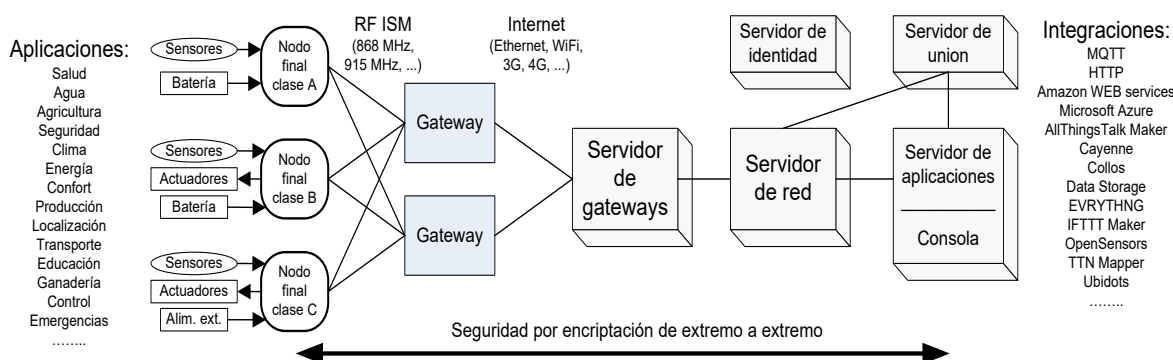
Figura 1. Ejemplo de arquitectura de red LoRAWAN.
