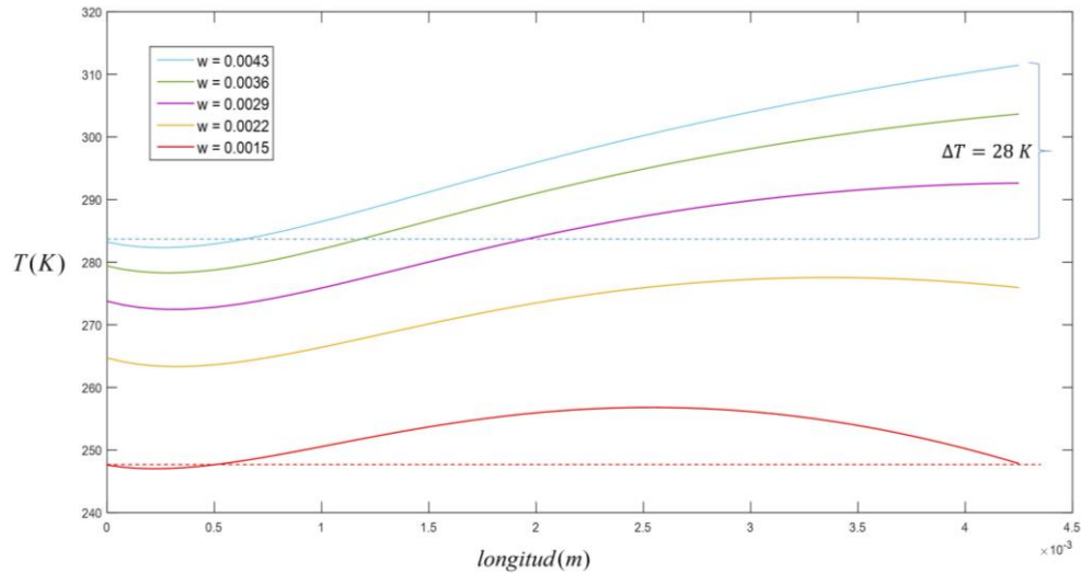
Figura 5. Perfiles espaciales de temperaturas a lo largo de la termocupla, para diferentes valores de w , durante el pulso de corriente eléctrica.
