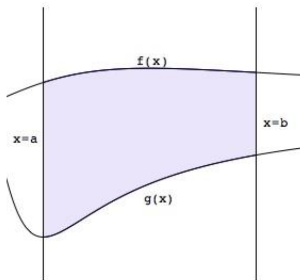
Figura 1. Región entre dos curvas cualesquiera.
