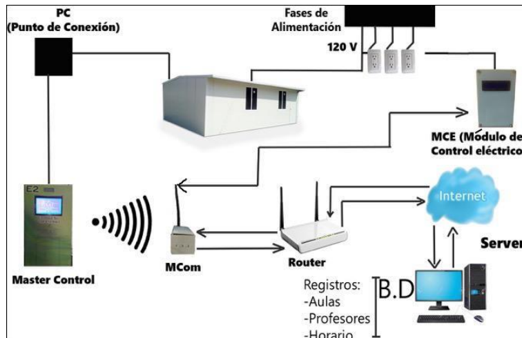
Figura 2. Componentes del Sistema de Administración Energética (SISAE), las flechas indican la comunicación entre los componentes. Funcionamiento del sistema
