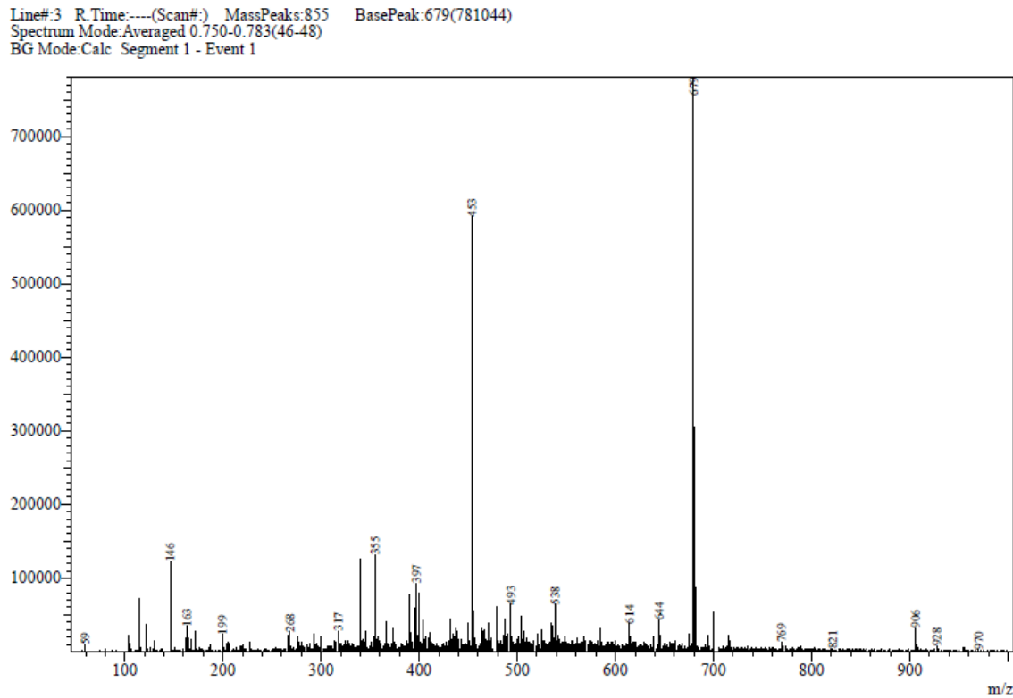
Figura 4: Cromatograma correspondiente al pico 3 del extracto metanólico de Syzygium aromaticum .
