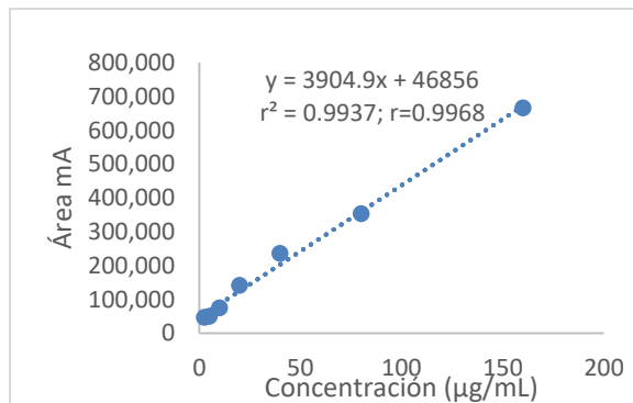
Figura 1. Gráfica de linealidad para DFC por el método de regresión lineal. Los resultados representan el \bar{X} \pm E.E de una n = 3 .
