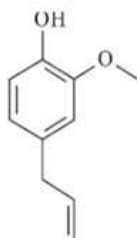
Figura 1. Estructura química del Eugenol (4-alil-2-metoxifenol). (González, 2002).
