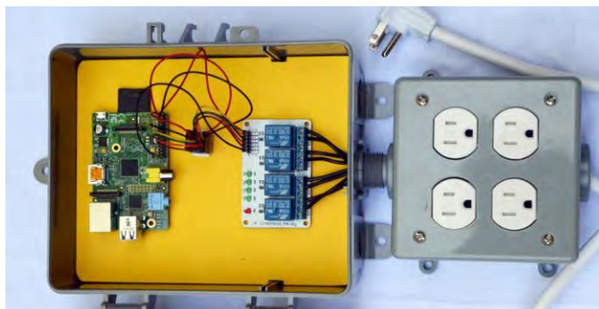
Figura 5: Raspberry Pi como medidor inteligente
