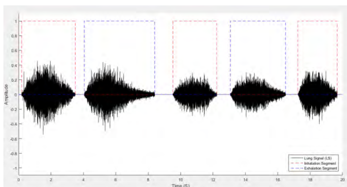
Figura 1. Segmentación automática sobre señales LS, aplicando VAD-GMM
