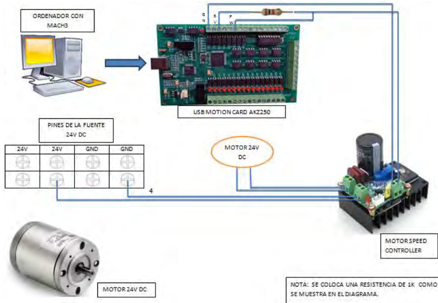
Figura 6. Circuito electrónico de conexión para el motor de CD para el husillo de la Fresadora CNC. CONFIGURACION DE MACH3
