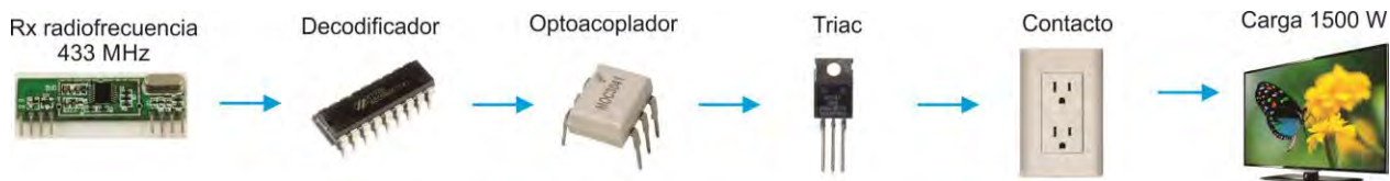
Figura 3. Diagrama a bloques del receptor.
