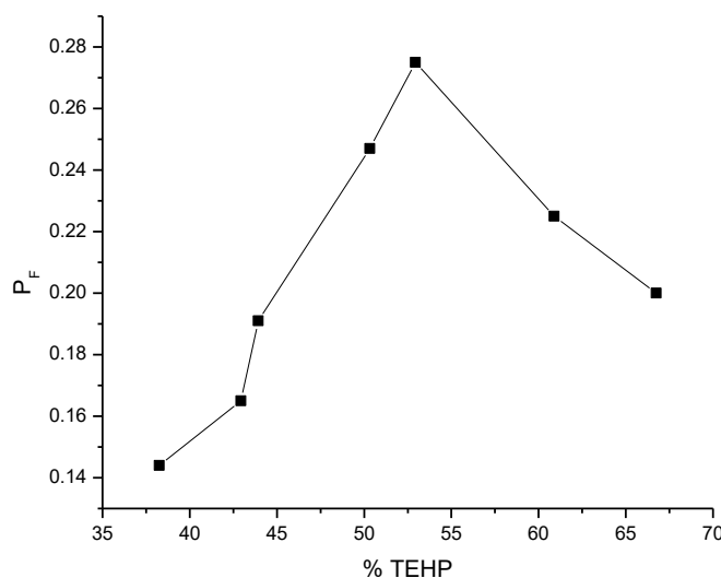
Figura 2. Variación de permeabilidad con respecto a la concentración del tris(2-etilhexil)fosfato para el transporte de oro a través de la membrana.
