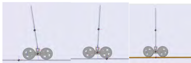
Figura 3. CAD del sistema de péndulo invertido.
