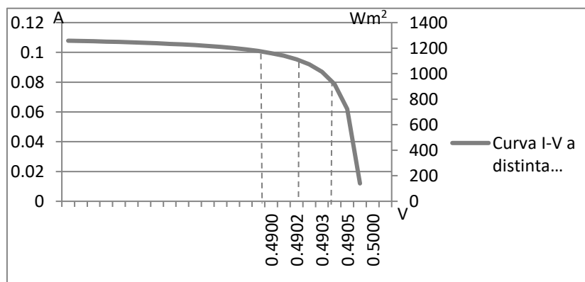
Figura 7 Curva I-V, a distinta irradiación y temperatura
