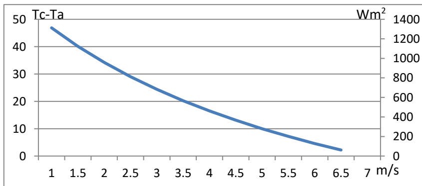
Figura 8 Relación del T_c - T_a , con respecto a la velocidad del viento y la irradiación solar teórica.
