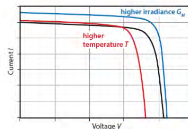
Figura 1 Curva de corriente y voltaje
