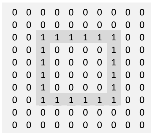
Figura 1. Cuadrado Binario
