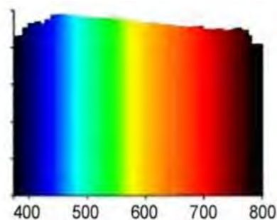
Fig. 2 Espectro Solar
