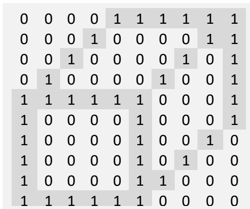
Figura 5. Cubo Binario
