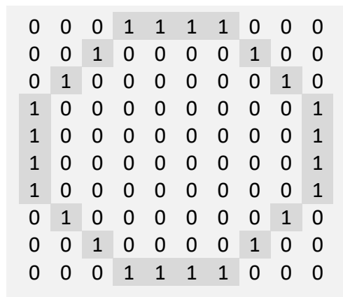
Figura 2. Círculo Binario
