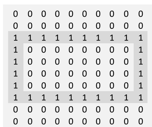
Figura 4. Rectángulo Binario
