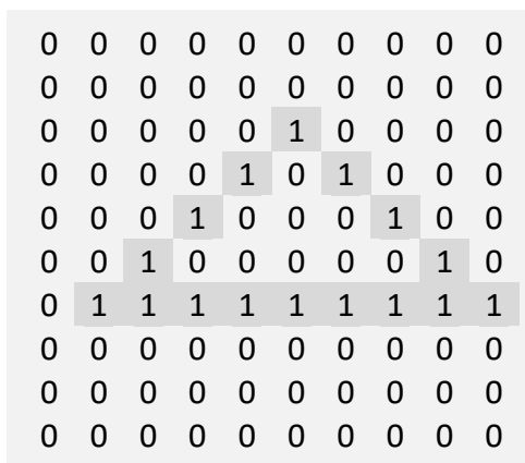
Figura 3. Triángulo Binario
