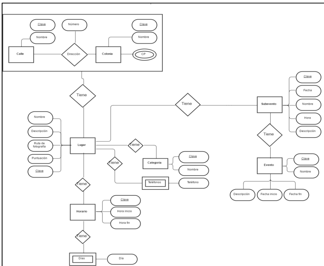
Figura 3. Diagrama Entidad-Relación
