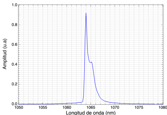
Figura 4. Longitud de onda de emisión del láser fabricado, ancho espectral de 1nm.
