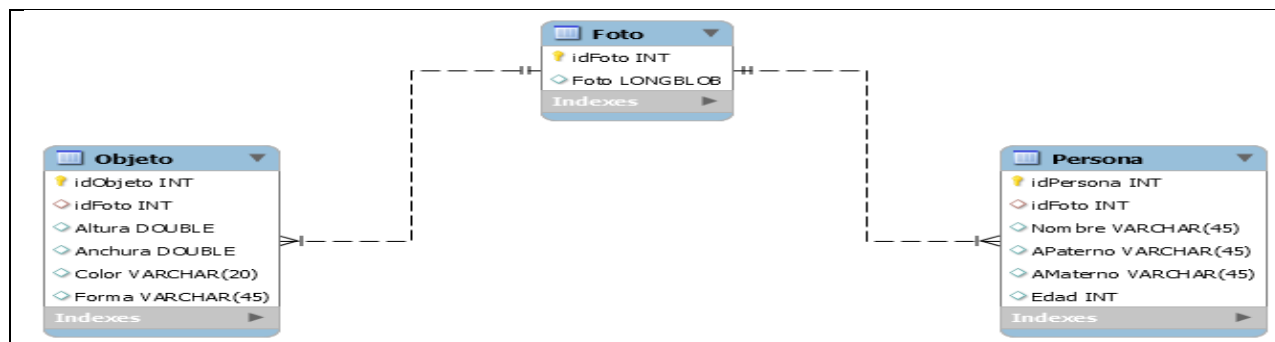
Figura 2. Modelo Entidad-Relación del Sistema de Base de Datos que almacena los objetos que son comparados con las imágenes que son captadas con el dron para terminar el reconocimiento de la persona.
