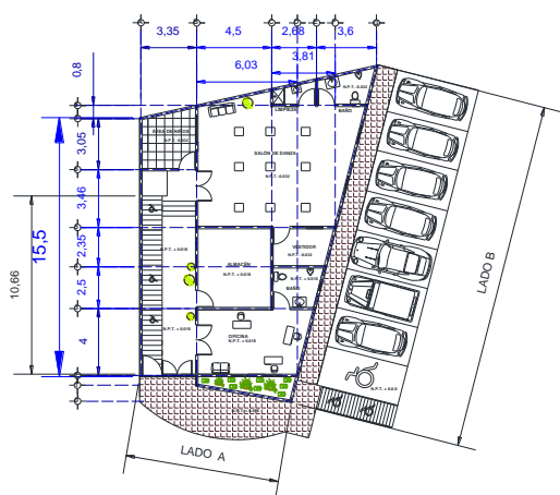
Figura 2. Primera propuesta en planta arquitectónica del área en estudio. Terreno ubicado Calle niño artillero por Casamata s/n, colonia El Polvorín, Ciudad de San Francisco de Campeche, Campeche, México. Fuente: Propia (2018)
