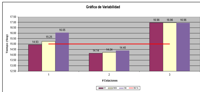
Figura 4. Tiempo ciclo de las estaciones de trabajo.
