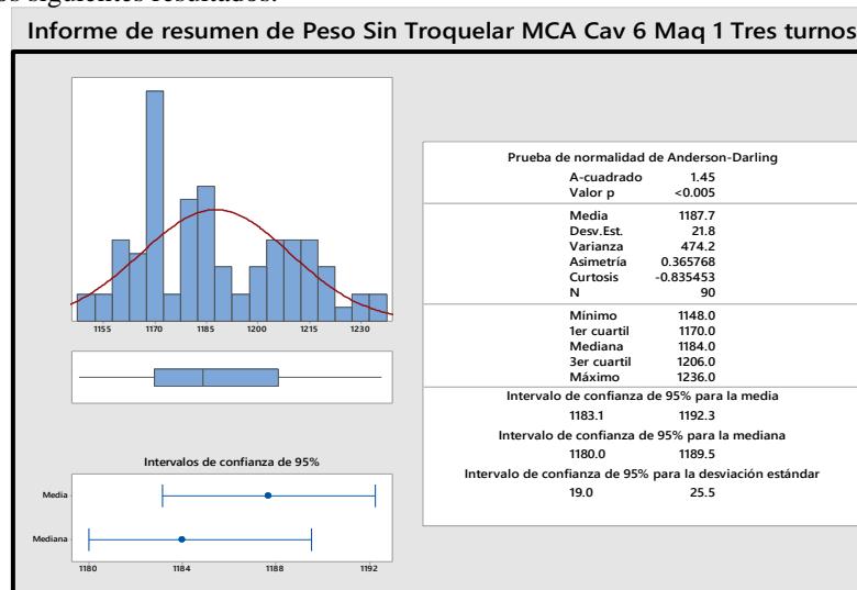
Figura 9. Pesos de las estructuras sin troquelar de la maquina 2
