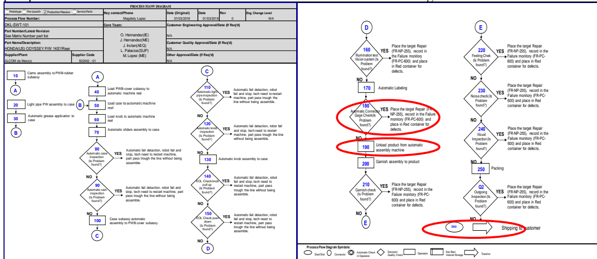
Figura 5. Diagrama de flujo de área de ensamble final
