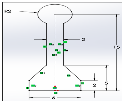
Figura 2. Perfil principal de la biela. Fuente: Diseño propio.
