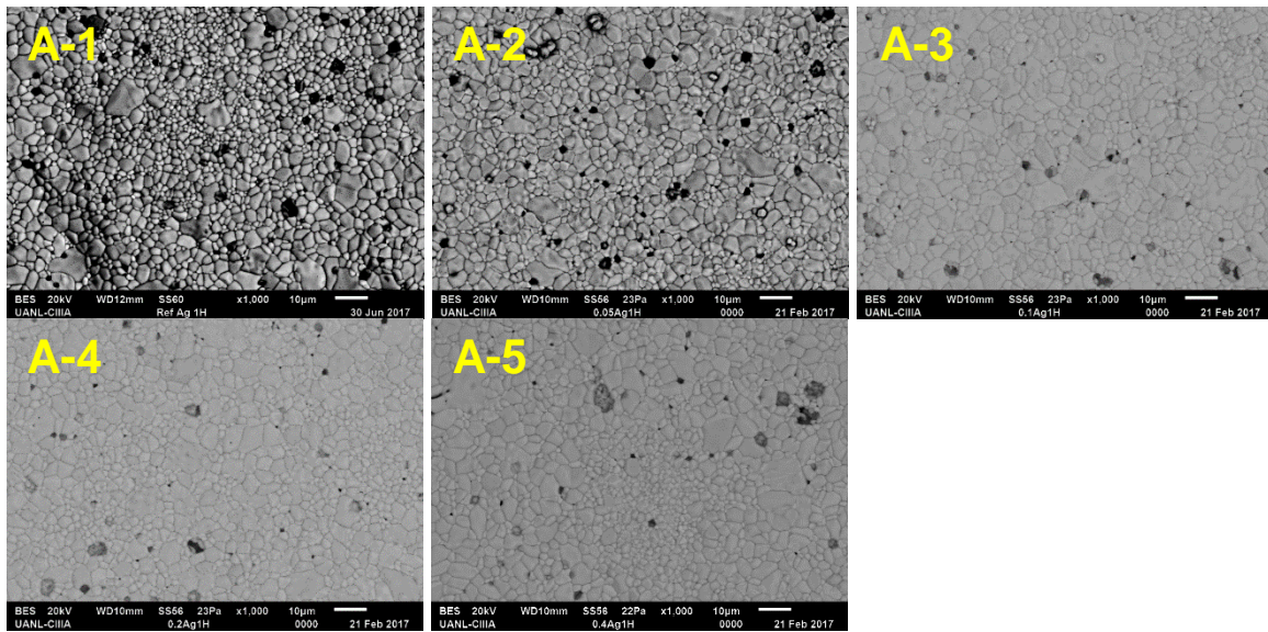
Figura 6 Imágenes de microscopía electrónica de barrido a 1,000 magnificaciones para las probetas experimentales con composición 98.95-X\%SnO_2 + 1.00\%Co_3O_4 + 0.05\%Ta_2O_5 + XAg , con diferentes contenidos de Ag en porcentaje molar: 1) Referencia, 2) 0.05%, 3) 0.10%, 4) 0.20%, 5) 0.40%. Donde los tiempos de sinterización son de A) 1hora,
