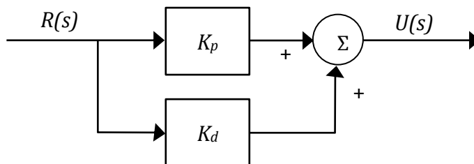
Figura 2. Control básico Proporcional Derivativo
