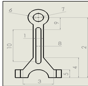
Figura 8. Guía de secuencia sugerida para medición de cotas funcionales (orden ascendente). Fuente: Diseño propio.
