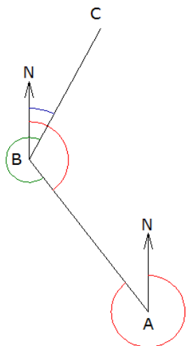
Figura 2. Gráfico de cálculo de distancias y azimut
