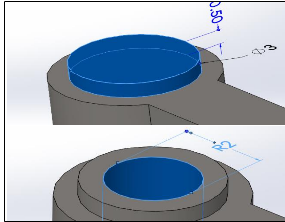
Figura 4. Detallado de la biela para unión con pistón. Fuente: Diseño propio.
