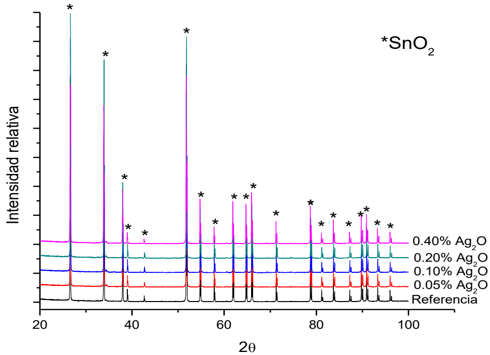
Figura 7 Patrones de DRX de las muestras en pastilla con diferentes concentraciones de Ag_2O , sinterizadas a 1350^{\circ}C durante 1 hora.
