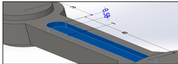
Figura 5. Detalle de corte. Fuente: Diseño propio.
