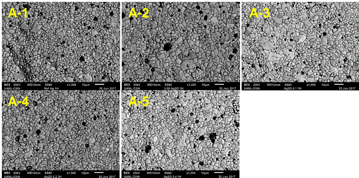
Figura 7 Imágenes de microscopía electrónica de barrido a 1,000 magnificaciones para las probetas experimentales con composición 98.95-X\%SnO_2 + 1.00\%Co_3O_4 + 0.05\%Ta_2O_5 + XAg_2O , con diferentes contenidos de Ag_2O en porcentaje molar: 1) Referencia, 2) 0.05%, 3) 0.10%, 4) 0.20%, 5) 0.40%. Tiempo de sinterización A) 1hora
