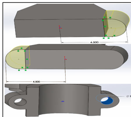
Figura 3. Formación y extrusión de montaje de contrabiela. Fuente: Diseño propio.
