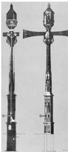
Figura 1 Diseño del semáforo de J.P. Knight.
