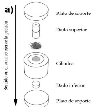
Figura 4 Molde.
