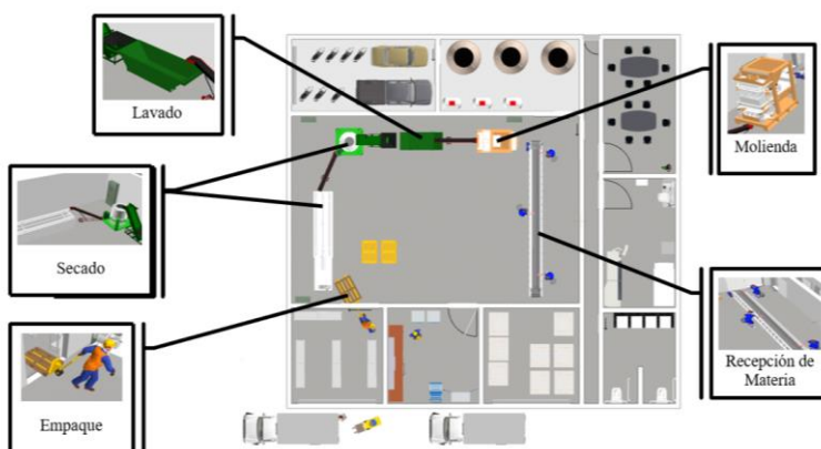
Imagen 2: distribución de planta y flujo del proceso
