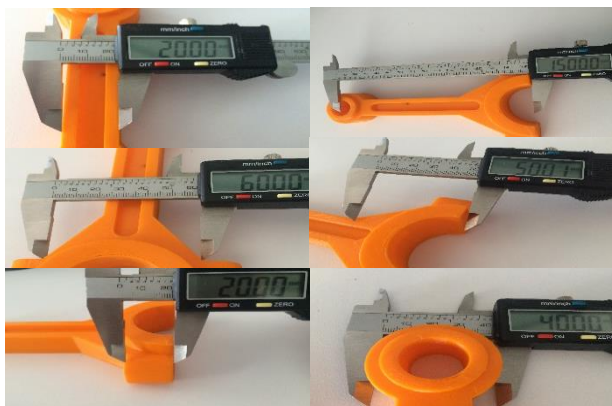
Figura 11. Procedimiento de Medición, paso 1 al 6. Fuente: Fotografías Propias.
