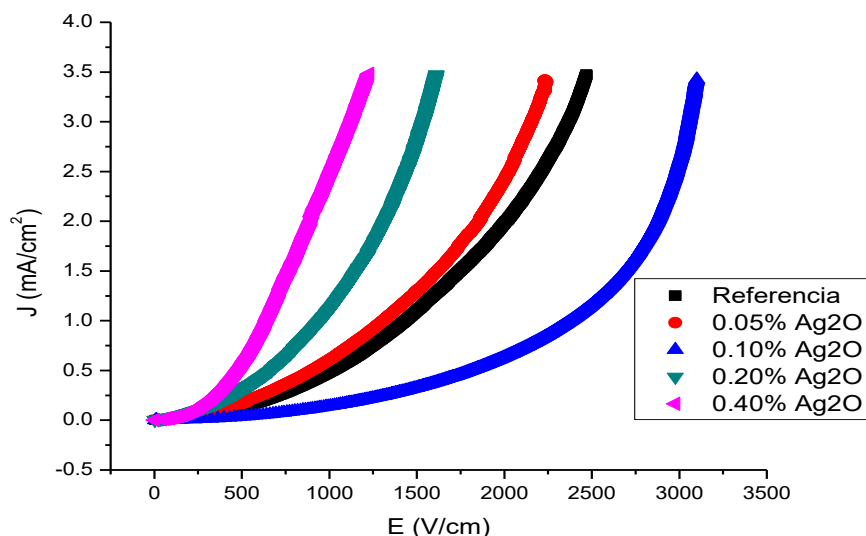
Figura 9 Grafica J-E de las muestras sinterizadas a 1350 °C por 1 hora con variación en el contenido de Ag 2 O.
