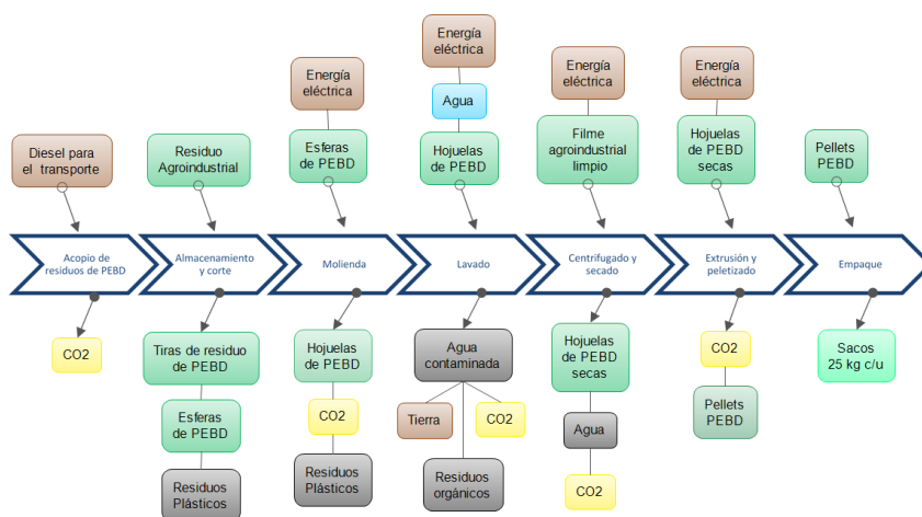
Diagrama 1: proceso de recuperación de residuos de PEBD
