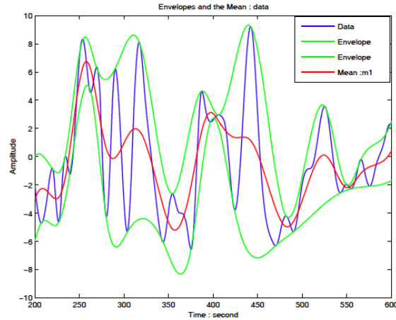
Figura 4. Comportamiento del filtrado de datos a través del EMD (Huang, Hilbert-Huang Transform and Its Applications, 2014)
