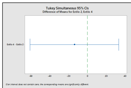
Figura 1.3 Grafica de intervalos de Tukey
