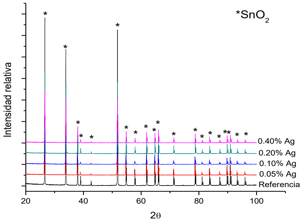
Figura 8 Patrones de DRX de las muestras en pastilla con diferentes concentraciones de Ag, sinterizadas a 1350°C durante 1 hora.
