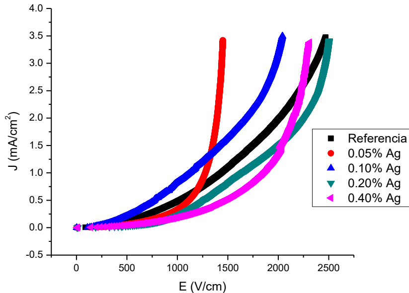
Figura 8 Grafica J-E de las muestras sinterizadas a 1350^{\circ}C por 1 hora con variación en el contenido de Ag.
