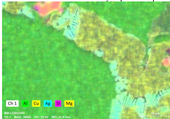
Análisis cualitativo en MEB muestra 3
