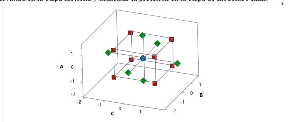
Figura 3 Esquema de Diseño Central Compuesto con tres factores, los niveles están señalados como -1, 0, 1.
