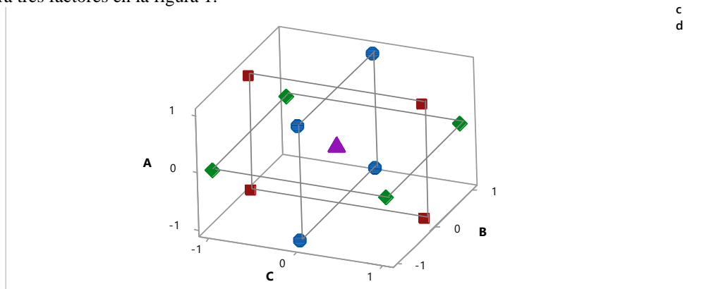
Figura 1 Esquema de arreglo Box-Behnken con tres factores, los niveles están señalados como -1, 0, 1.
