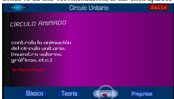
Figura 8. Círculo Unitario
