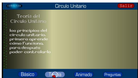
Figura 5. Círculo Unitario
