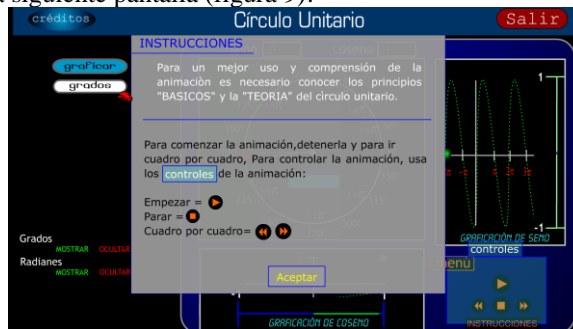
Figura 9. Recomendación
