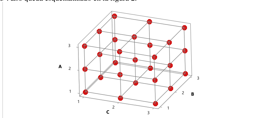
Figura 2 Esquema de arreglo L27 con tres factores ( 3^3 ). Con niveles 1, 2 y 3.
