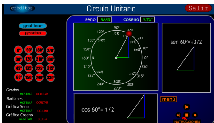
Figura 11. Ángulo Especial
