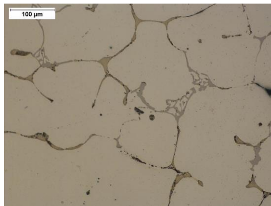
Aleación rica en Cu modificada con Ag, 200x muestra 13
