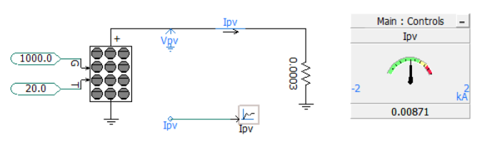
Fig. 6. Simulando para un valor de R_s = 0.0003 \Omega
