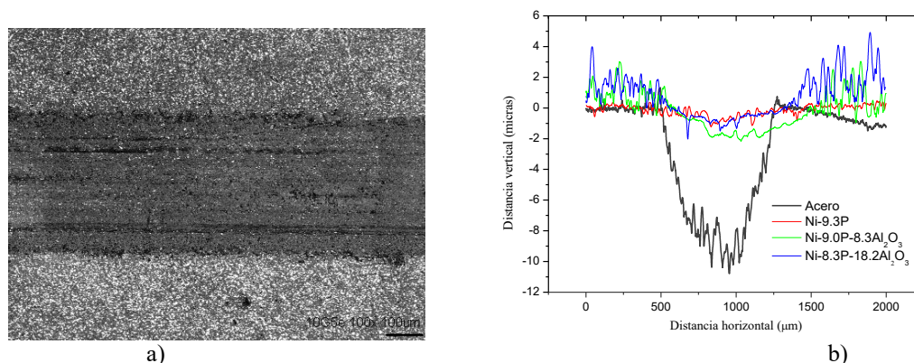
Figura 6 Huella de desgaste del depósito Ni-8.3P-18.2Al 2 O 3 a: (a) 10N y (b) Perfiles observados de la huella de desgaste de los diferentes depósitos a 5N.
