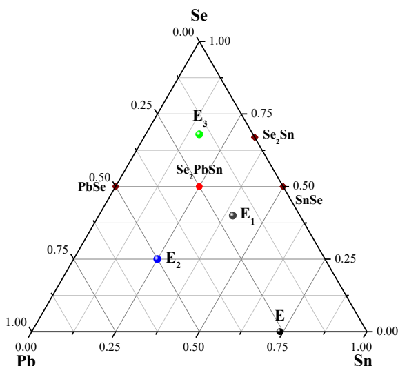
Figura 1. Representación esquemática del sistema Pb–Sn–Se. Los vértices representan los elementos puros.
