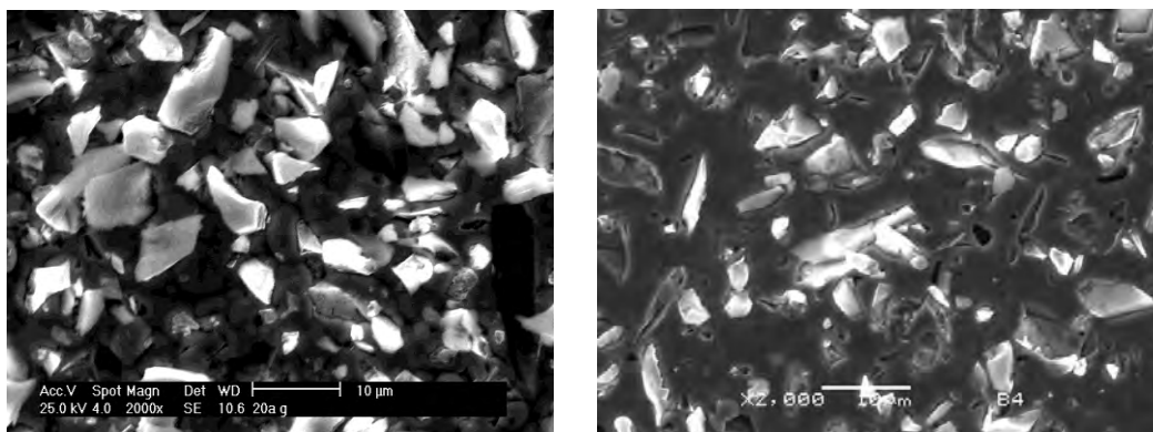
Figure 2. Imágenes SEM de los recubrimientos Ni-P-Al 2 O 3 de (a) sin tratamiento térmico y (b) Tratado térmicamente
