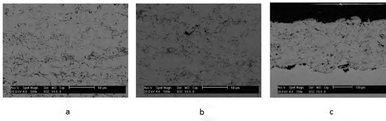
Figura 5 Microestructura de la sección transversal del recubrimiento a) 5 cm b) 10 cm c) Partículas contaminantes.
