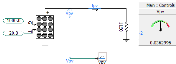
Fig. 5. Simulando para un valor de R_{sh} = 1160 \Omega
