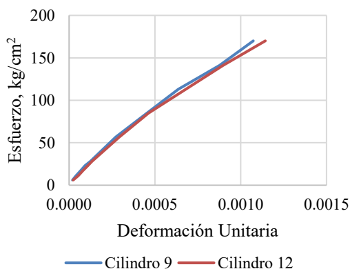
Figura 7. Gráfica Esfuerzo-Deformación de la prueba de módulo de elasticidad a los 28 días
