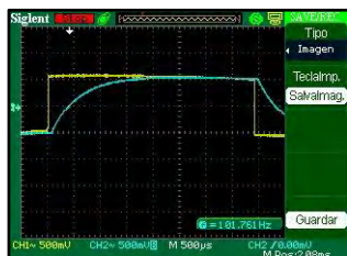
Fig 5. Observación experimental de sistema de primer orden
