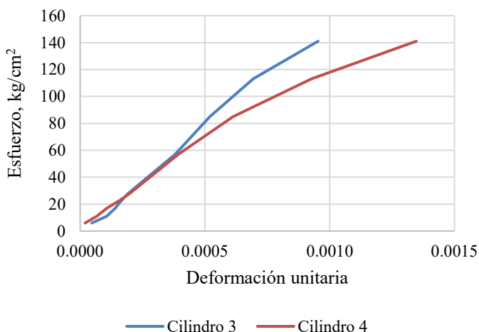
Figura 5. Gráfica Esfuerzo-Deformación de la prueba de módulo de elasticidad a los 7 días.
