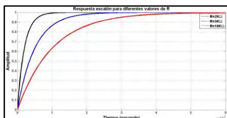
Fig 7. Simulación de la función de transferencia para diferentes valores de R ( R = 2K\Omega, 5K\Omega, 10K\Omega ).
