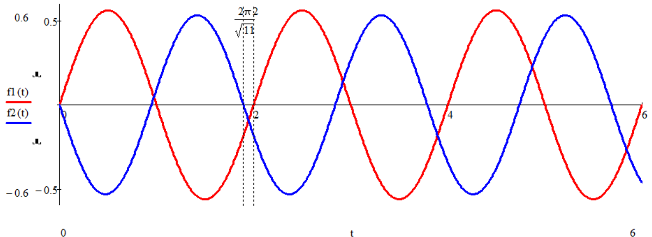
Figura 4: Gráfica de las funciones que definen la respuesta del sistema en cuasiresonancia: La función f_1(t) (en rojo) y la f_2(t) (en azul) coinciden en el punto (0, 0): La roja después de 2 segundos regresa a x = 0 y la azul lo hace después de 2\pi/\sqrt{11} segundos: ¿Cuál es el tiempo t_1 en el que coinciden por primera vez en el punto x = 0 ; ( t_1, 0 )?
