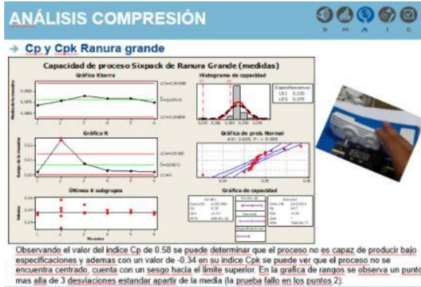
Figura 2. Medición de desempeño del proceso.
