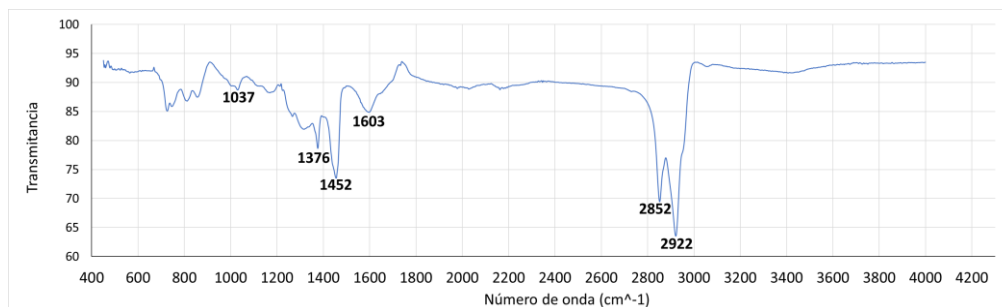
Figura 5. Espectro FTIR de los Asfaltenos.
