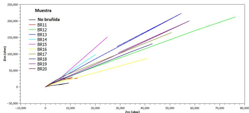
Figura 5. Curvas de Tafel para las muestras BRT11-BRT20.
