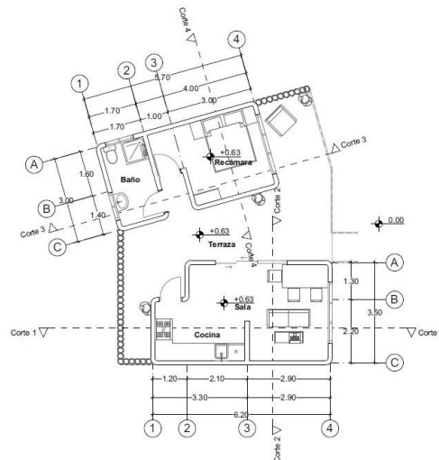
Figura 1. Plano Arquitectónico 66.84 M 2 . Elaboración Propia
