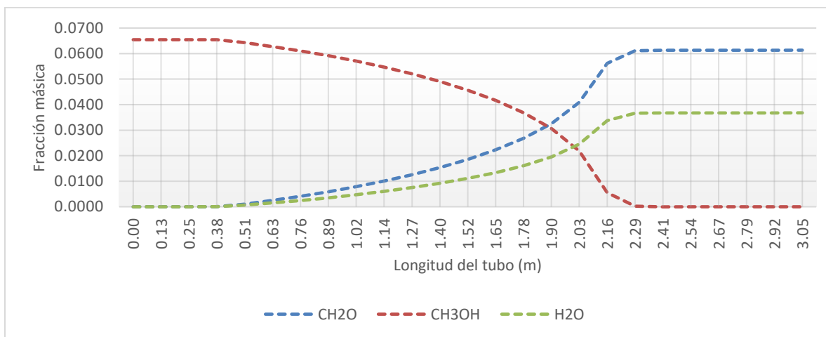
Figura 2. Producción de formaldehído con catalizador a 5 m/s.
