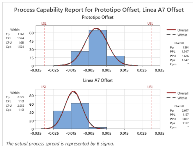
Figura 3. Análisis estadístico de repetibilidad del sistema de posicionamiento de herramental.
