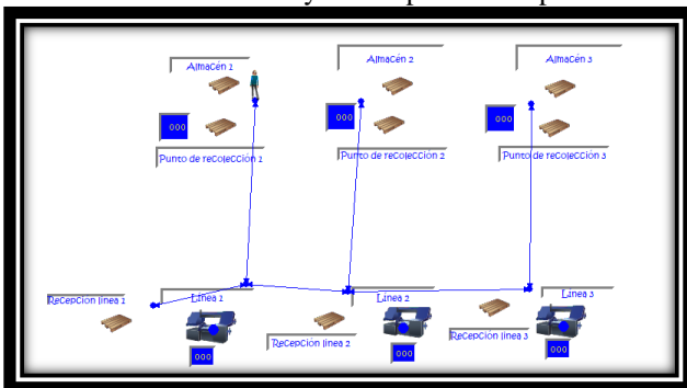
Figura 1. Layout del proceso productivo del sistema convencional.
