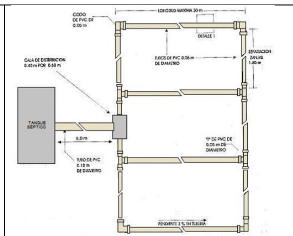
Figura 2. Tubería distribuida en paralelo (CNA, 1994).
