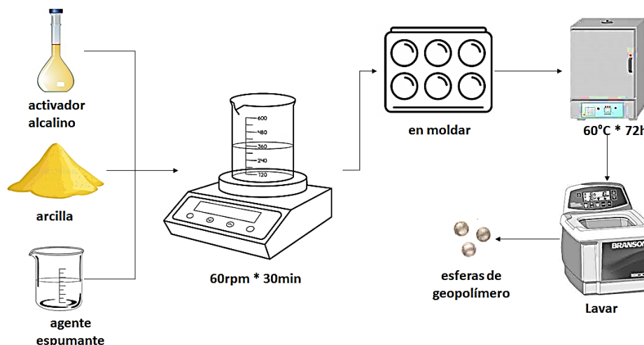
Figura 1. Método de síntesis de geopolímeros porosos.
