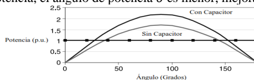
Figura 1.0 Transferencia de potencia de una línea de transmisión sin y con compensación capacitiva.
