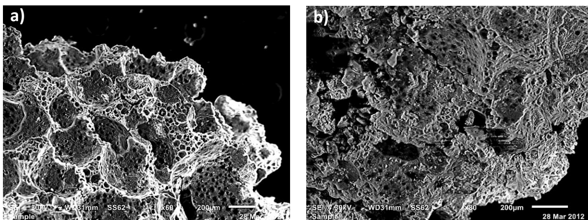
Figura 3. (a) Microestructura de poros del geopolímero 2.4. (b) Microestructura de poros del geopolímero después de la remoción de Cromo.
