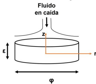
Figura 1. Descripción del sistema analizado y EDP con condiciones de frontera e iniciales
