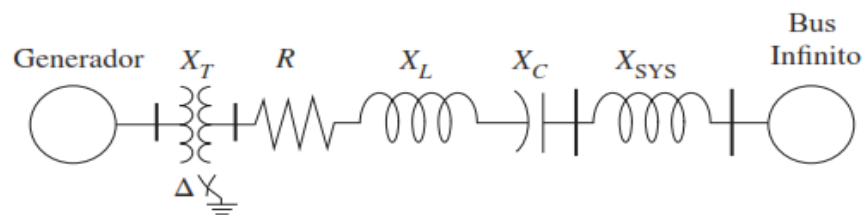
Figura 2.0. Primer Modelo de Referencia de la IEEE.
