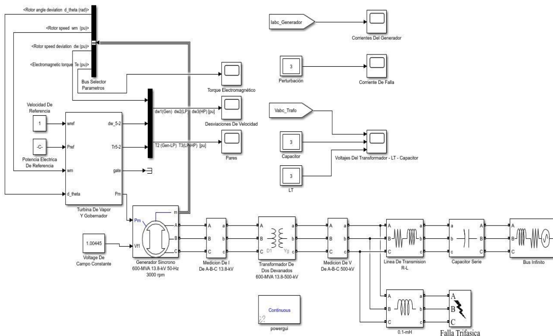
Figura 4.0. Simulación del Primer Sistema de Referencia de la IEEE para observar la amplificación de pares.
