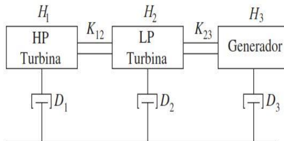
Figura 3.0. Representación física del sistema Turbina – Generador.
