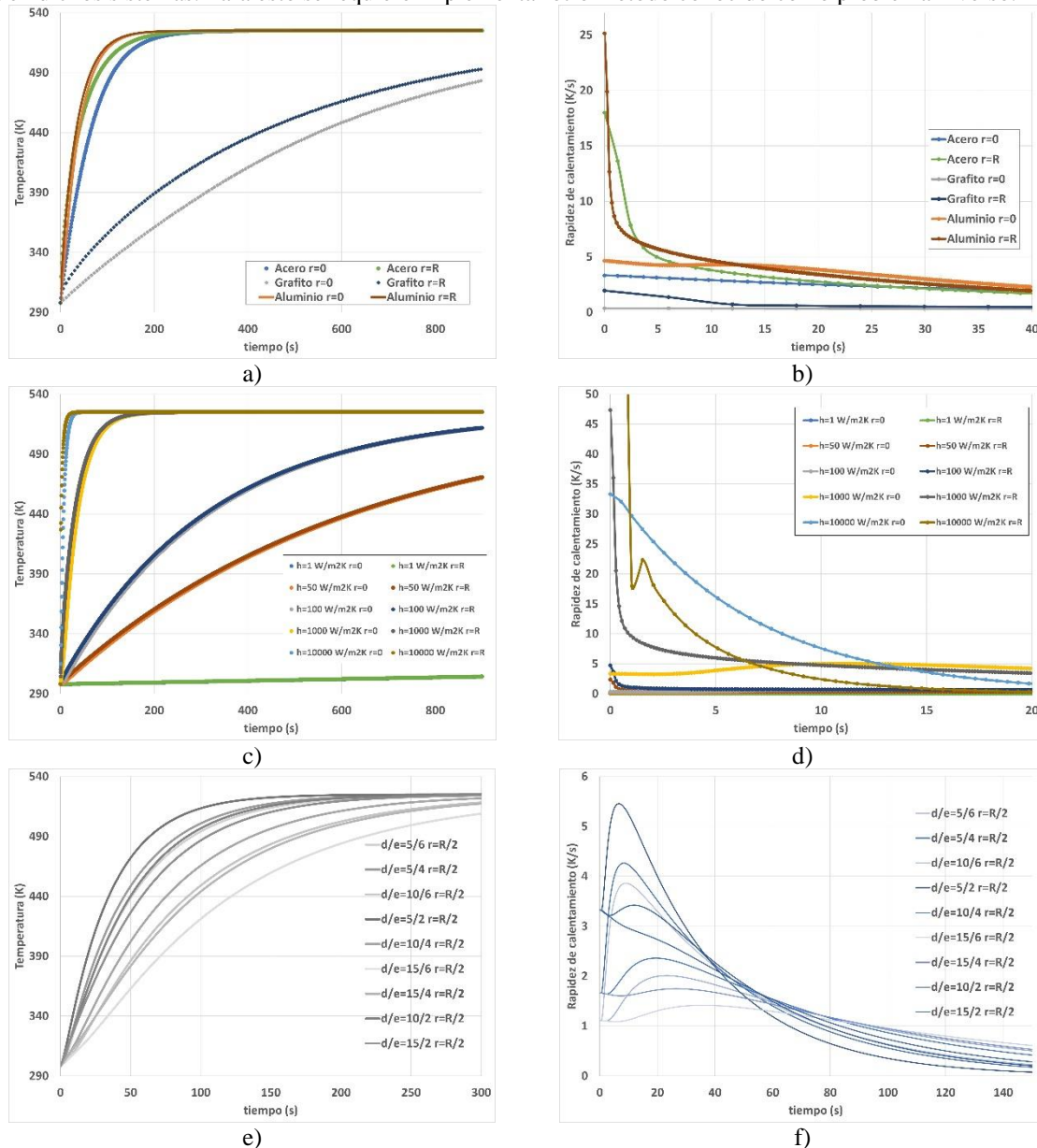
Figura 2. Efecto sobre el perfil de temperatura en el cilindro de: a) Tipo de material; c) Coeficiente de convección; e) Relación \phi/\epsilon . Efecto sobre la rapidez de calentamiento de: b) Tipo de material; d) Coeficiente de convección; f) Relación \phi/\epsilon .
