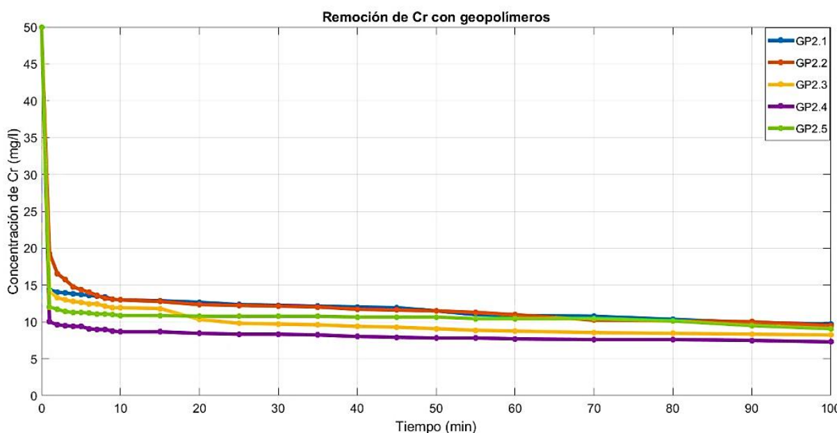
Figura 2. Remoción de Cr con geopolímeros.
