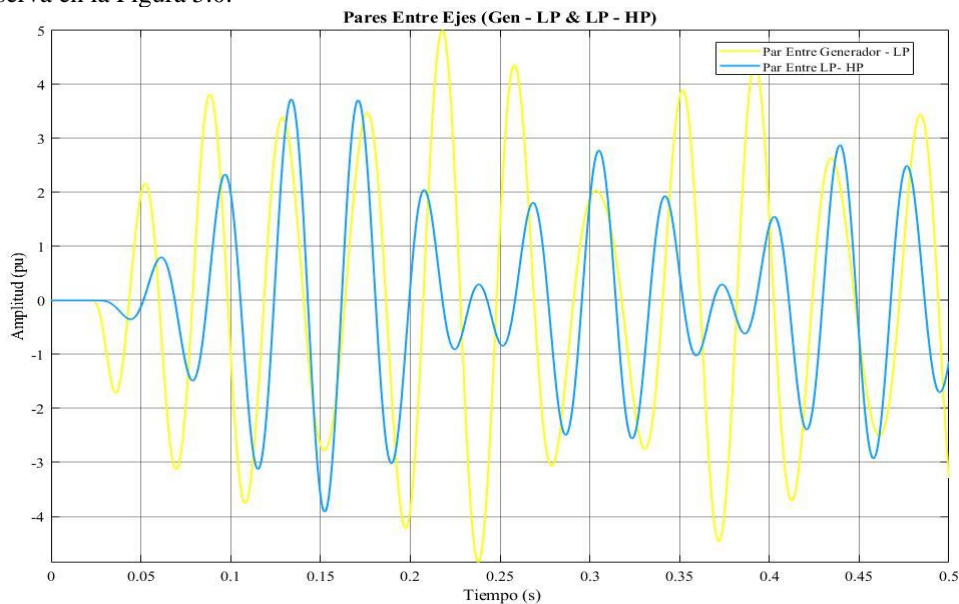
Figura 5.0. Pares del sistema Turbina – Generador.
