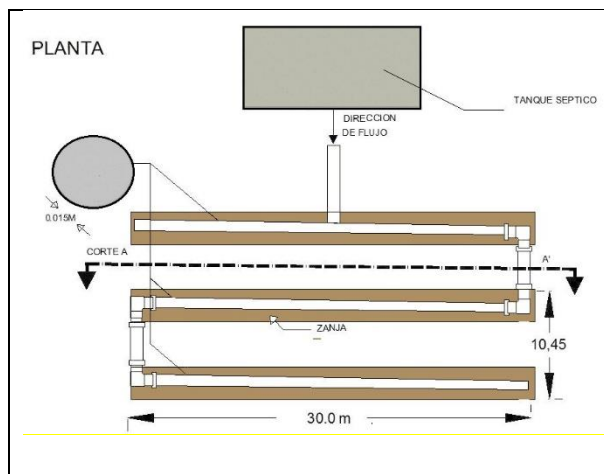
Figura 1. Tubería de distribución en serie (CNA, 1994).
