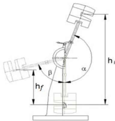
Figura 1. Variables físicas en el péndulo de impacto
