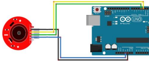
Figura 4. Esquema de conexión encoder- tarjeta de adquisición de datos
