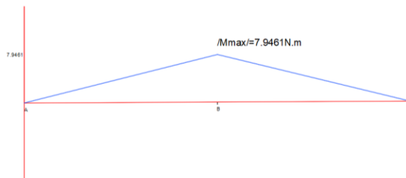
Figura 6 Diagrama de momento flexionante
