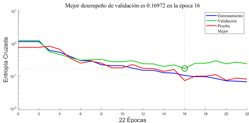
Figura 3 Entrenamiento de la red neuronal.
