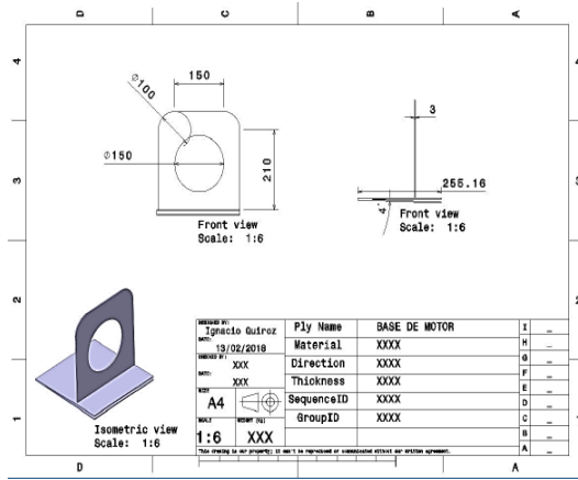
Figura 7 Base del motor
