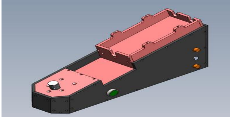
Figura 7. Prototipo del ensamble de ABS negro para sujeción del Chatillon del dispositivo pull tester
