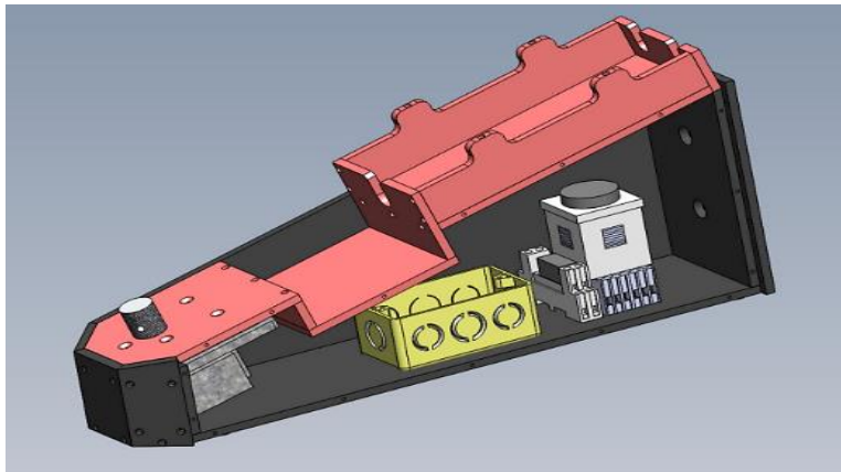
Figura 8. Parte interna del ensamble de ABS negro con componentes electrónicos
