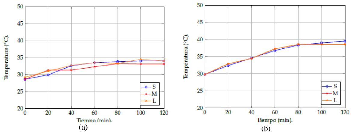
Figura 4. Temperatura medida en los tres piezoeléctricos de prueba L=113 KHz, M=1.7MHz, S=2.5MHz a) en el depósito de agua, b) en el medio de vapor de agua
