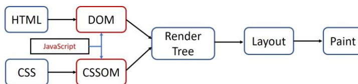
Figura 1. Estructura de una página Web de procesamiento del navegador. Fuente Grigoriak, 2013.
