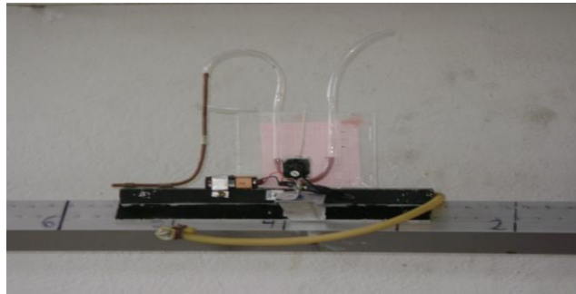
Figura 6. Riel Levitador para calibración de tubos Pitot
