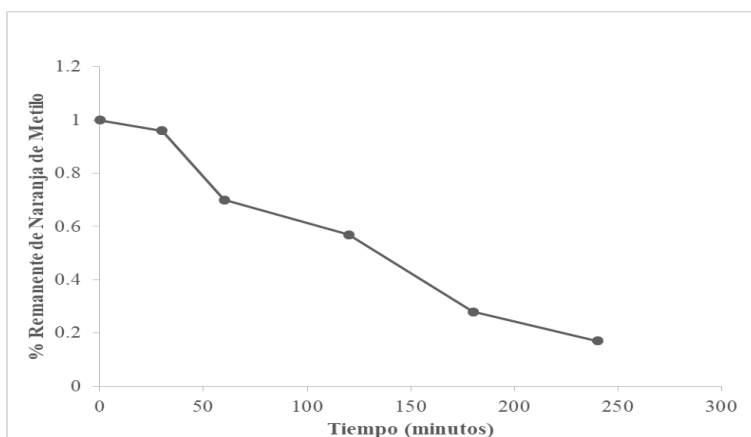
Figura 1. Perfil de decoloración fotocatalítica de Naranja de Metilo (10 ppm).
