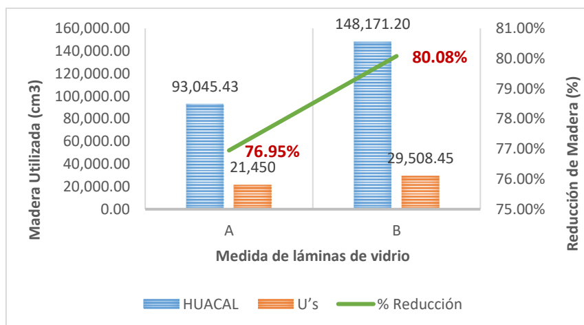
Gráfica 4 - Comparación de reducción de madera utilizada en empaques
