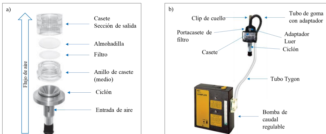
Figura 1. Tren de muestreo. a) Ensamble de casete de filtro con ciclón. b) Tren de muestreo final.
