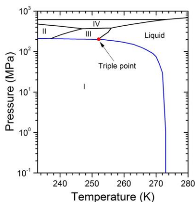
Figura 1. Diagrama de fase para la preservación isocórica (Angulo-Sherman & Mercado-Uribe, 2014)
