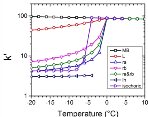
Figura 2. Comparación de las constantes dieléctricas del experimento con capacitor (Angulo-Sherman, 2019)
