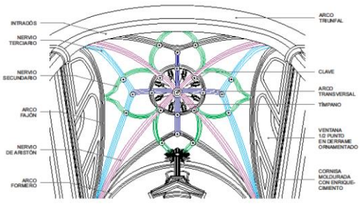
Figura 26. Bóveda de Cruería en Ábside
