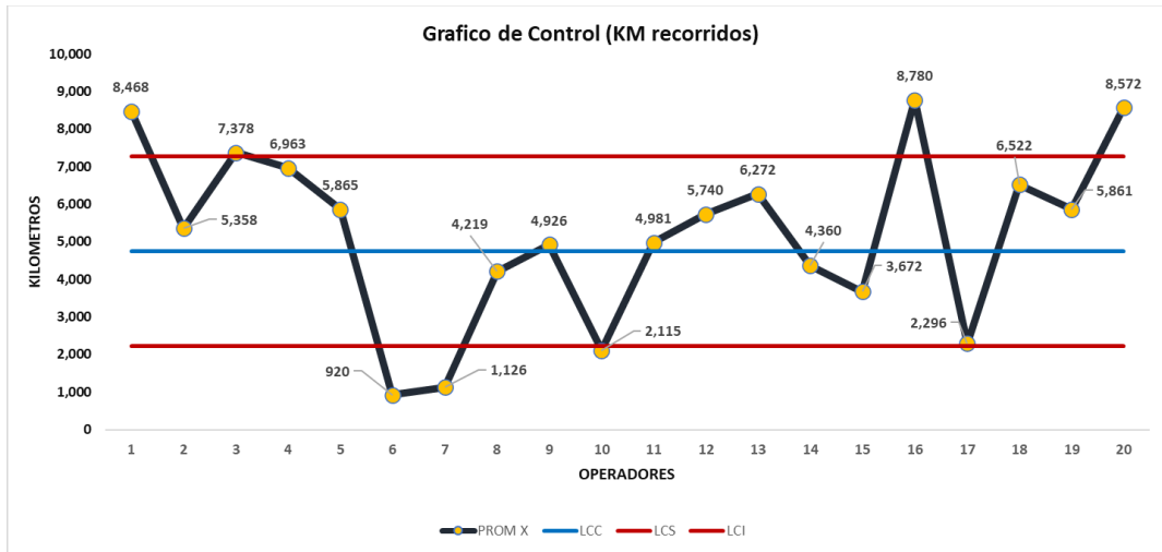
Figura 4. Gráfico de control de kilómetros recorridos.
