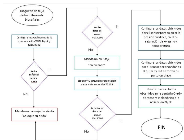
Figura 3. Diagrama de flujo del programa para monitoreo de bioseñales
