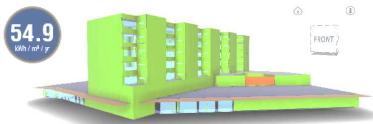
Figura 4. Modelo energético definitivo del hospital geriátrico en Insight 360.
