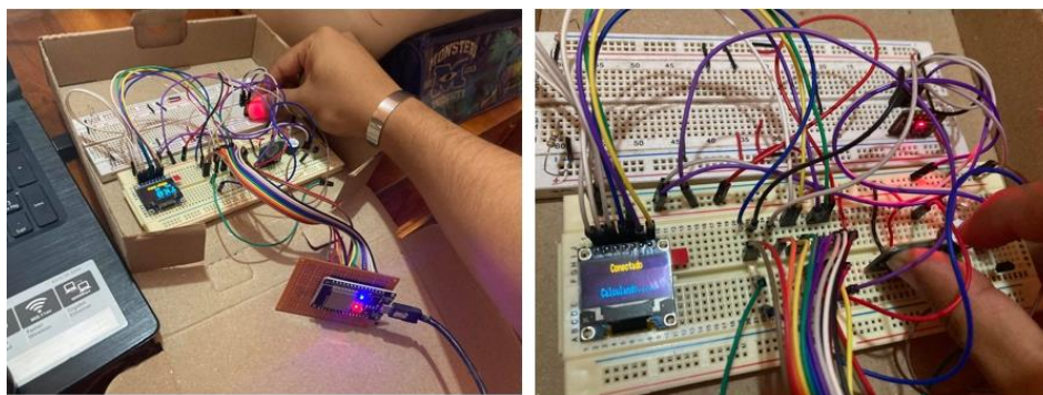
Figura 5 Implementación de circuito para el monitoreo de bioseñales
