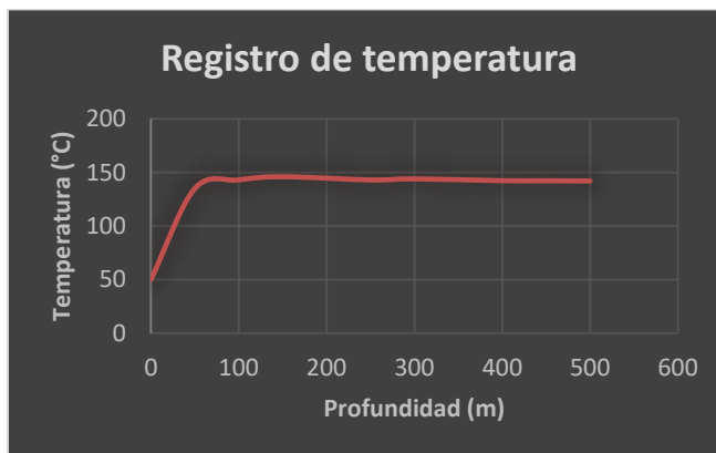
Figura 4. Registro de temperatura del pozo geotérmico.
