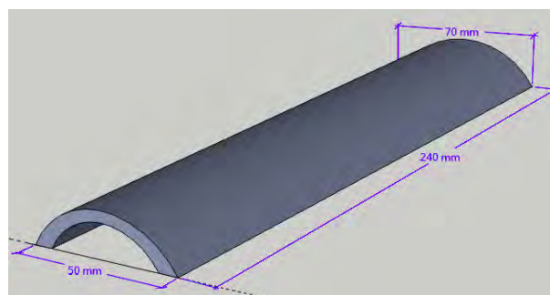
Figura 7: Dimensiones de la teja de plástico
