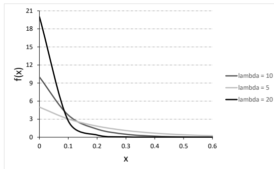
Figura 2. Forma de la Distribución Exponencial con diferentes tasas
