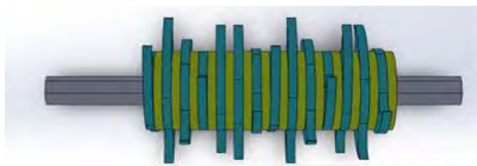
Figura 2. Configuración de cuchillas para el proyecto.
