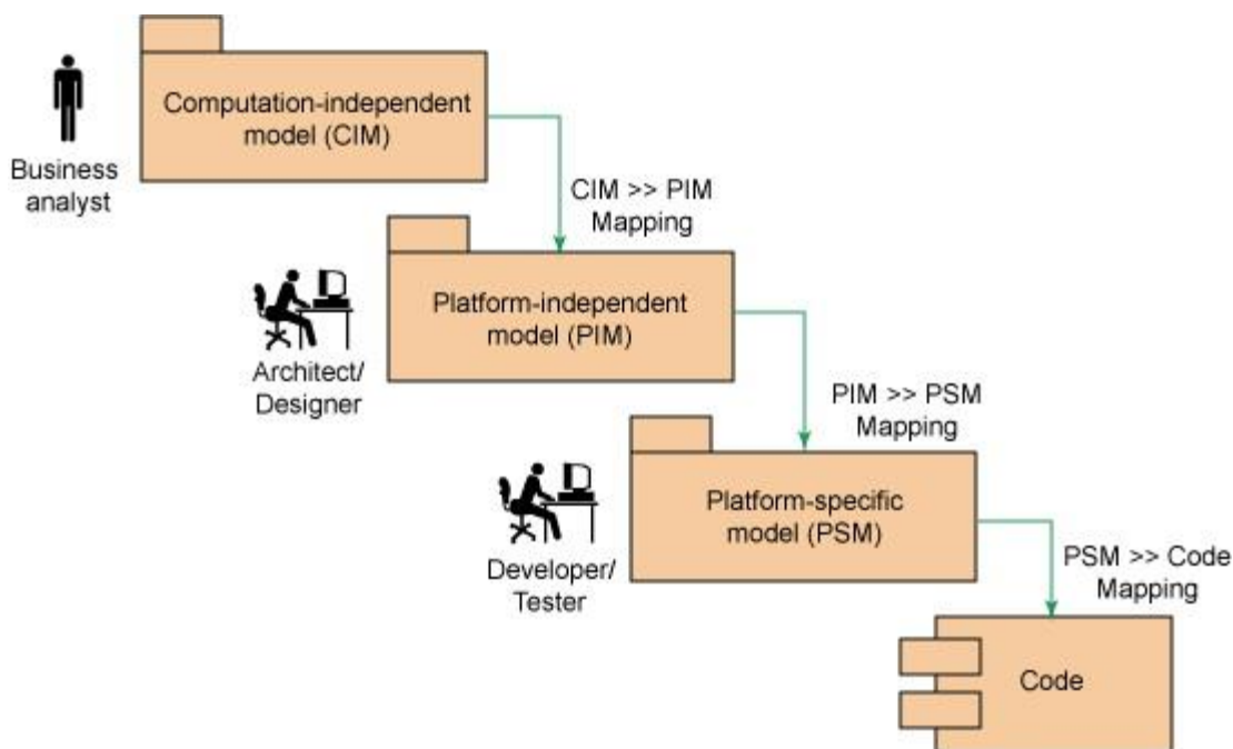
Figura 1. Ingeniería Dirigida por Modelos.
