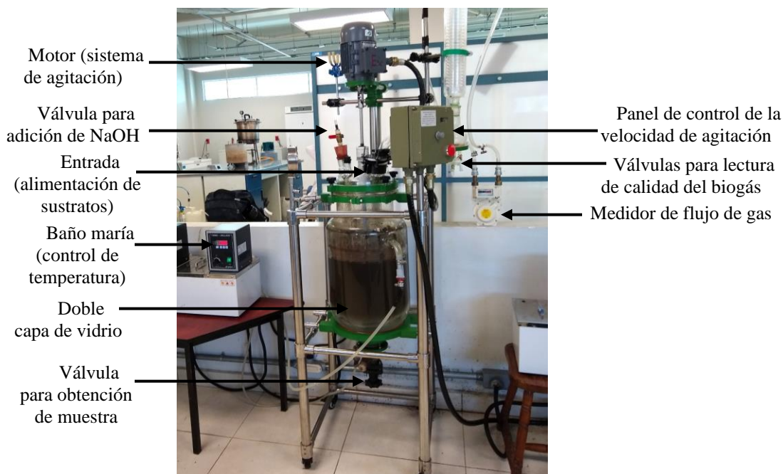
Figura 1. Biorreactor anaerobio CSTR y sus componentes principales.
