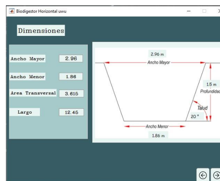
Figura 7. Dimensiones de la zanja del biodigestor. Fuente: Elaboración propia (2022).
