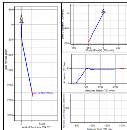
Figura 3. Seguimiento direccional del pozo.
