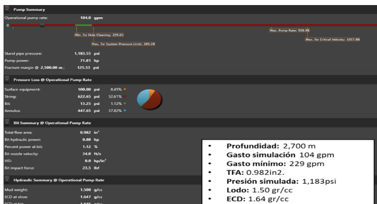
Figura 6. Análisis de hidráulica.
