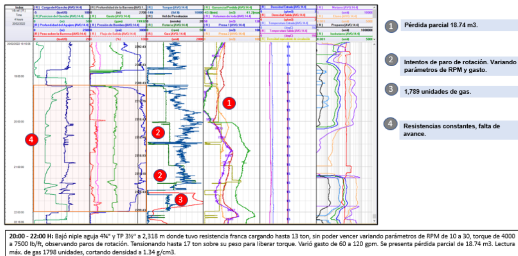
Figura 7. Alerta operativa de evento durante la perforación.
