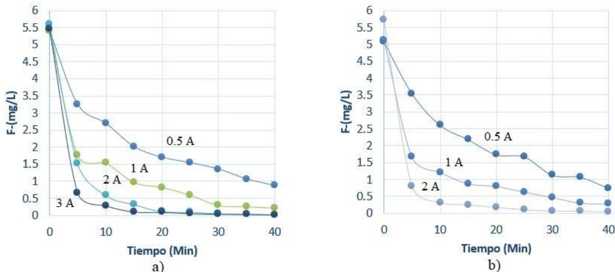
Figura 2. Variación de la concentración de flúor respecto al tiempo de EC bajo la adición de: a) NaCl grado reactivo; y, b) NaCl comercial.
