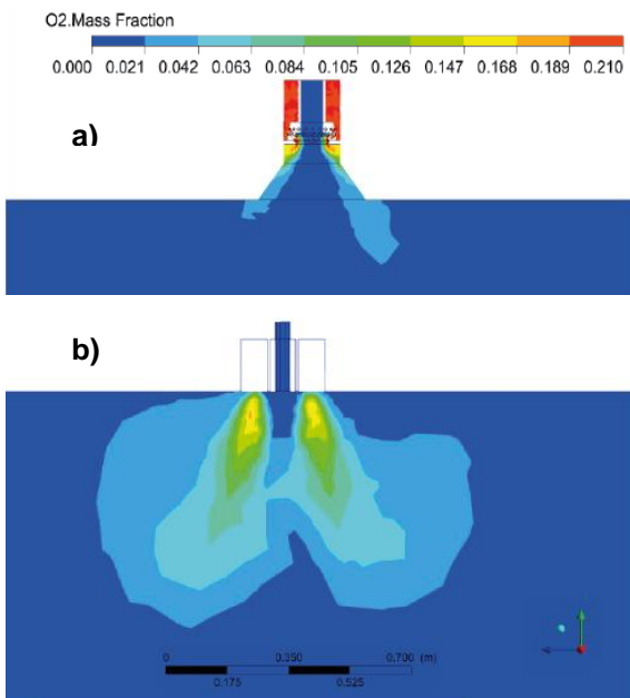
Figura 6. Contorno de la Fracción de masa del Oxígeno libre en el volumen interno de la cámara de combustión: caso 1 (a), y caso 2 (b).
