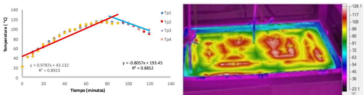
Fig.7.- Variación de la temperatura durante el calentamiento y el enfriamiento del aceite con respecto al tiempo, con sus respectivas líneas de tendencia, imagen de la distribución de la energía calorífica con las temperaturas en 6 puntos
