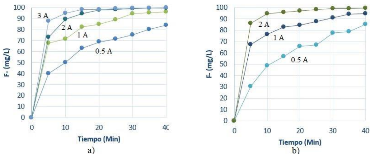
Figura 3. Variación del % de remoción de flúor respecto al tiempo de EC bajo la adición de: a) NaCl grado reactivo b) NaCl comercial
