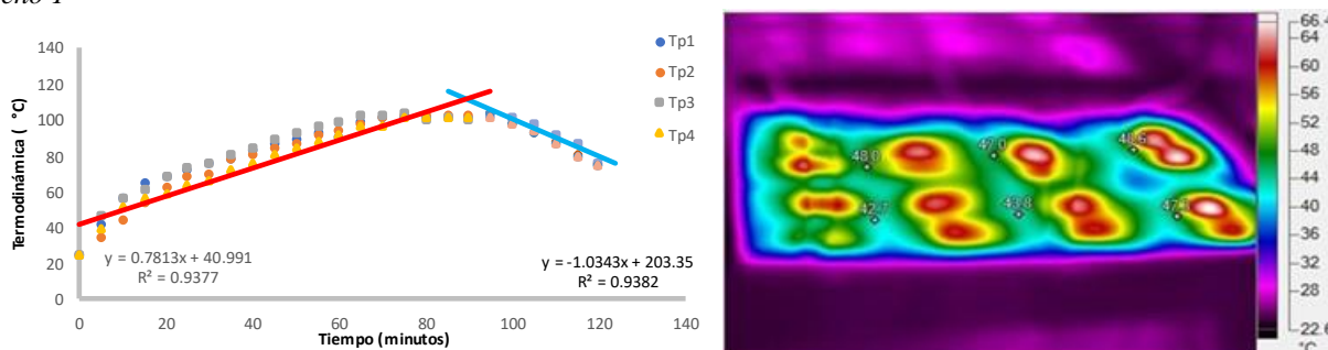
Fig. 4.- Variación de la temperatura durante el calentamiento y el enfriamiento del aceite con respecto al tiempo, con sus respectivas líneas de tendencia, imagen de la distribución de la energía calorífica con las temperaturas en 6 puntos.
