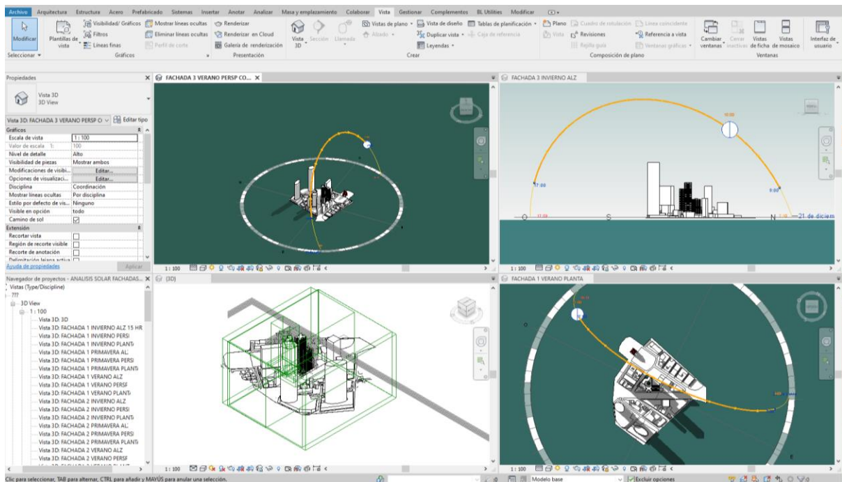
Figura 3. Edificios multifuncionales: se trabajó el Estudio de Asoleamiento en un modelo LOD200, año 2019, haciendo uso de la metodología BIM en una fase específica de proyecto: Análisis.
