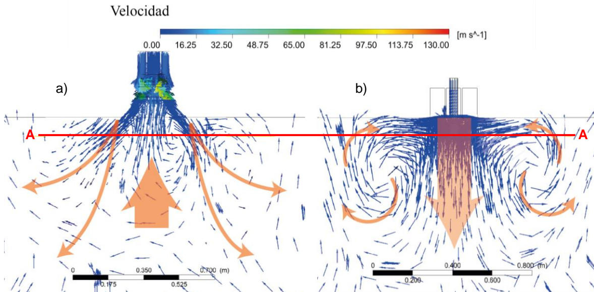
Figura 4. Vectores de velocidad en la sección transversal: caso 1 (a), y caso 2 (b).
