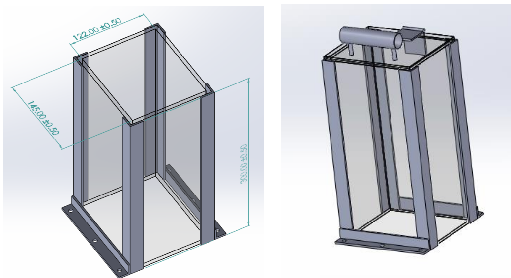
Figura 5. Dimensiones de la tolva (izquierda) y tolva con compuerta (derecha)
