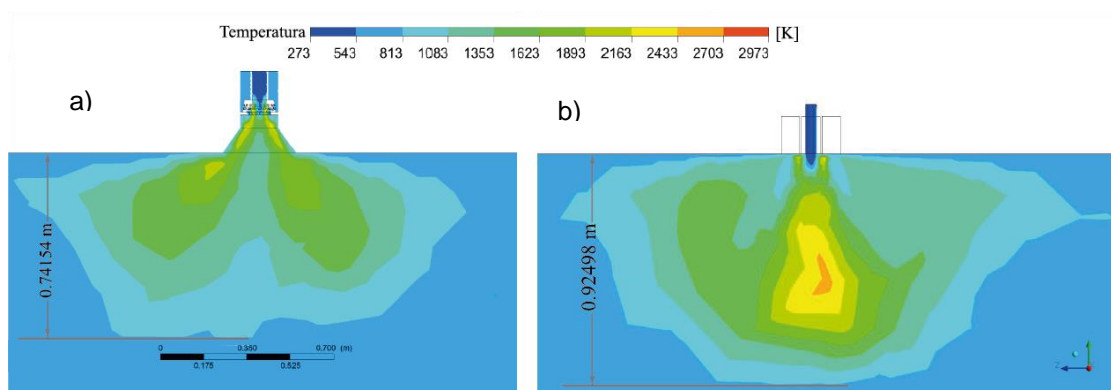
Figura 3. Perfiles térmicos con longitud de flama a los 5 segundos: caso 1 (a), y caso 2 (b).
