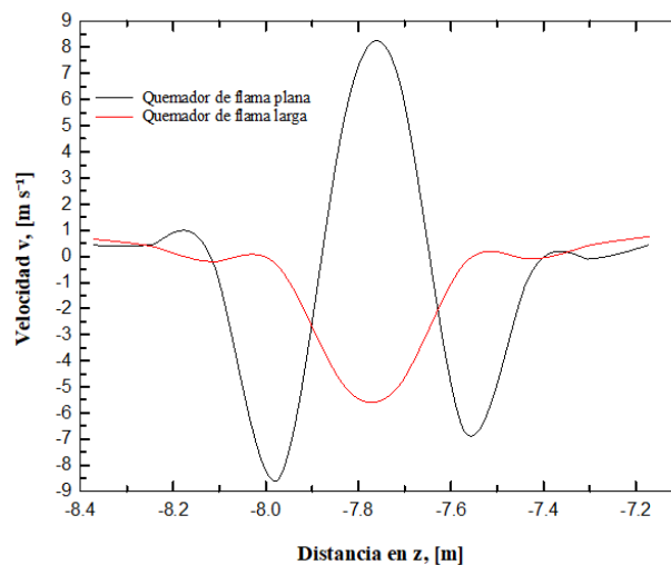
Figura 1. Magnitud de la componente Y de la velocidad sobre la línea A
