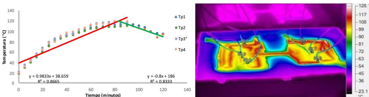
Fig. 5.-Variación de la temperatura durante el calentamiento y el enfriamiento del aceite con respecto al tiempo, con sus respectivas líneas de tendencia, imagen de la distribución de la energía calorífica con las temperaturas en 6 puntos
