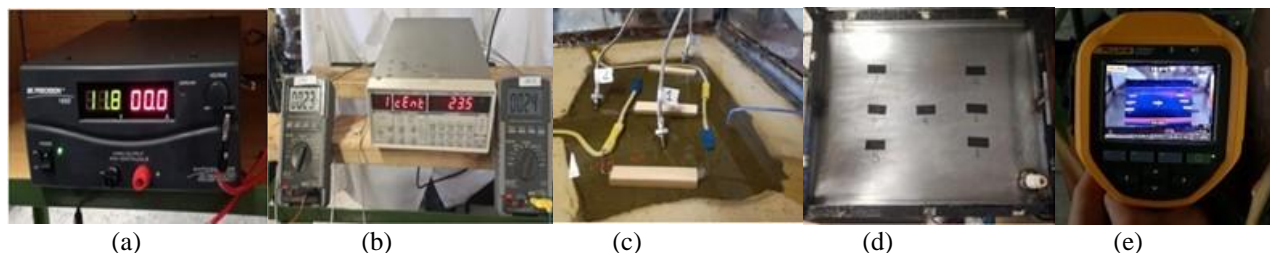
Figura 3.- (a) fuente de poder de corriente directa, (b) sistema de registro de temperaturas, (c) termopares tipo k, (d) colocación de cinta negra en los puntos en los que se determina la temperatura en la superficie de cocción, (e) Imagen de la cámara termográfica.
