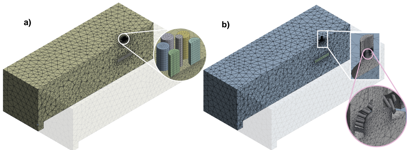
Figura 1. Malla computacional: caso 1, quemador de flama plana (b) y caso 2, quemador de flama larga (a).
