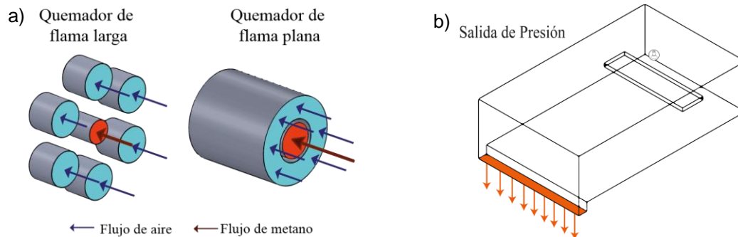
Figura 2. Ubicación de las condiciones frontera de entrada de flujo másico (a) y salida de presión (b).
