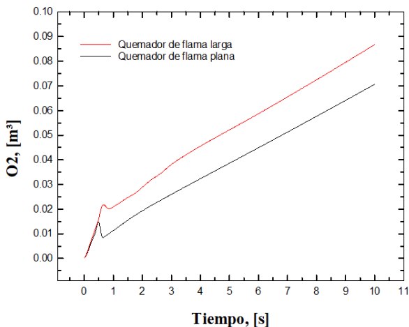
Figura 7. Fracción másica del oxígeno libre en el volumen de la cámara de combustión a lo largo del tiempo
