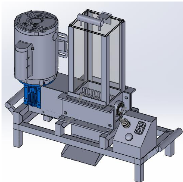
Figura 6. Ensamble de máquina trituradora con tolva.
