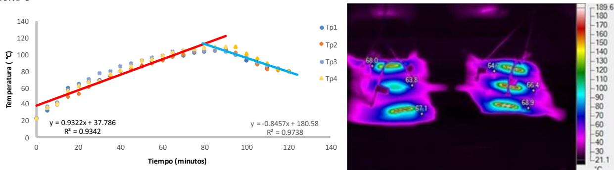
Fig. 6- Variación de la temperatura durante el calentamiento y el enfriamiento del aceite con respecto al tiempo, con sus respectivas líneas de tendencia, imagen de la distribución de la energía calorífica con las temperaturas en 6 puntos
