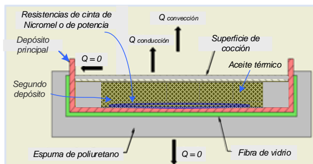
Fig. 1 Vista lateral del almacén de aceite térmico
