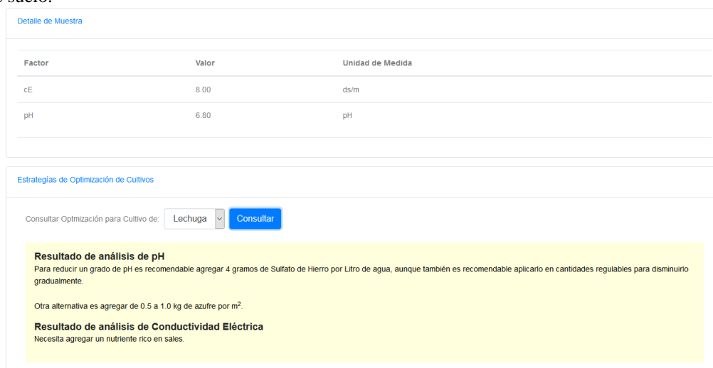
Figura 5. Sección de la interfaz de usuario que ayuda a determinar la estrategia de tratamiento del suelo tomando como base los valores de los factores pH y CE de una muestra de suelo para el cultivo de Lechuga.
