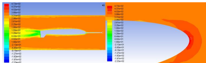
Figura 8. a) Perfil de presión, b) acercamiento a la nariz del tubo Pitot donde incide P_{m\acute{a}xima}
