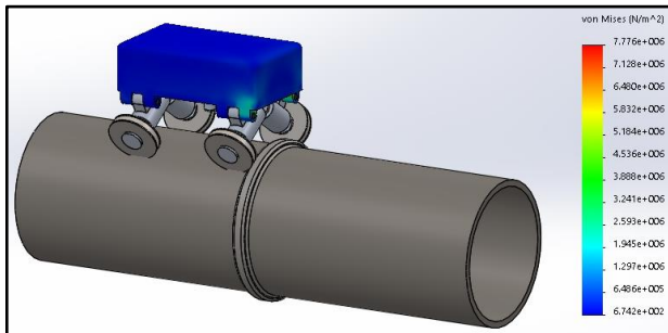
Ilustración 9 Simulación dinámica
