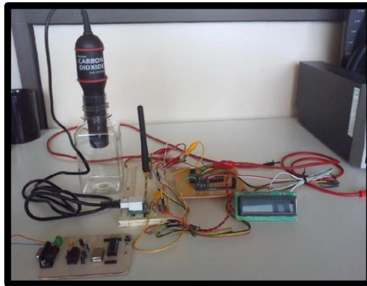
Figura 3. Tarjetas y sensores del sistema de comunicación inalámbrica.
