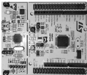
Figura 1. Tarjeta de desarrollo NUCLEO-L476RG.
