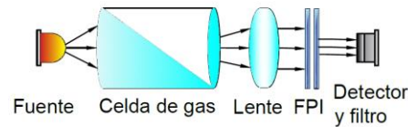
Figura 2. Arreglo experimental propuesto para la utilización del método MGFPI para la detección del SF_6
