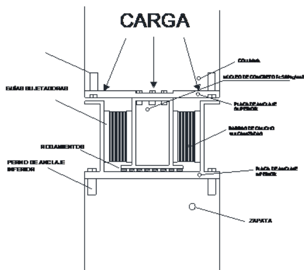
Figura 4. Prototipo inicial con rodamientos y amortiguador lateral de caucho reciclado. Fuente: Elaboración propia
